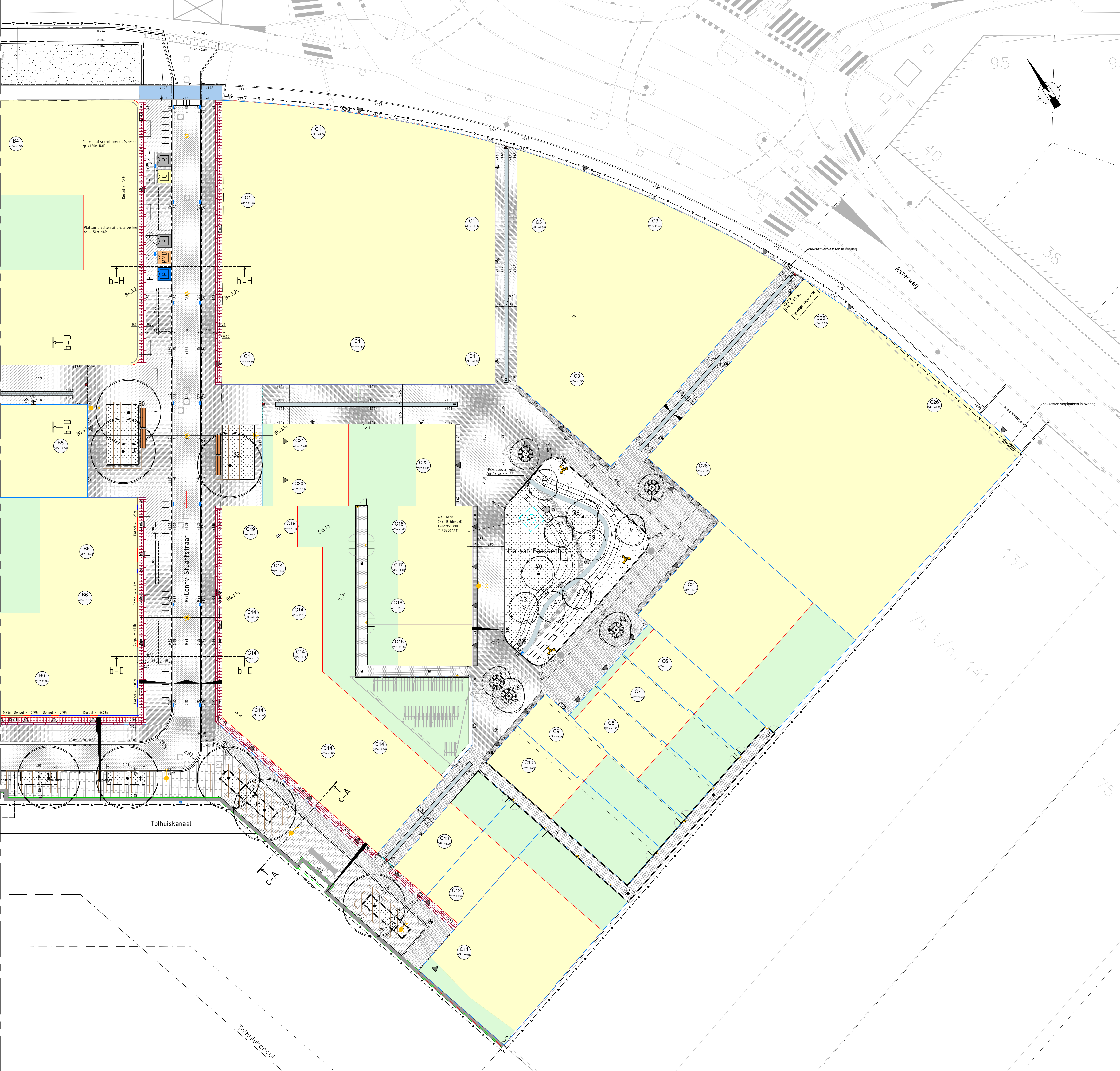
Inrichtingstekening bouwblok C schaal 1:200
