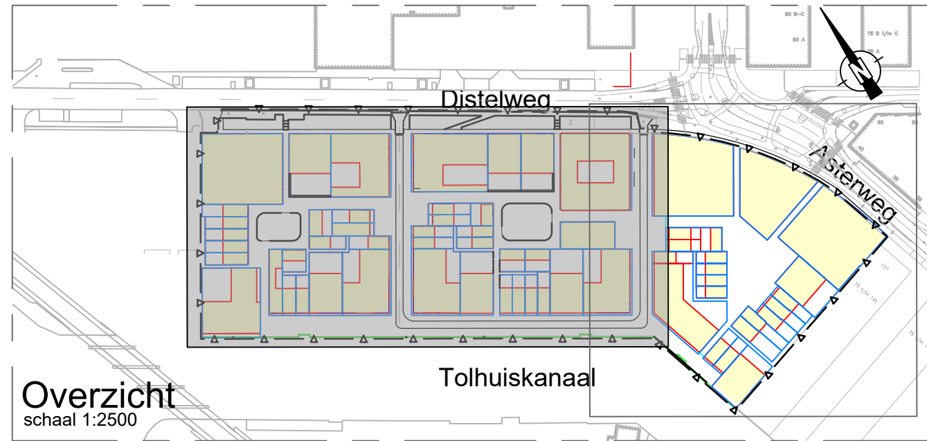
Overzicht schaal 1:2500
