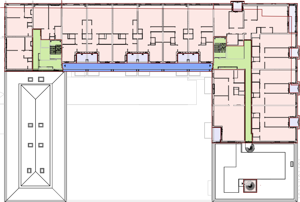
05 vijfde verdieping
