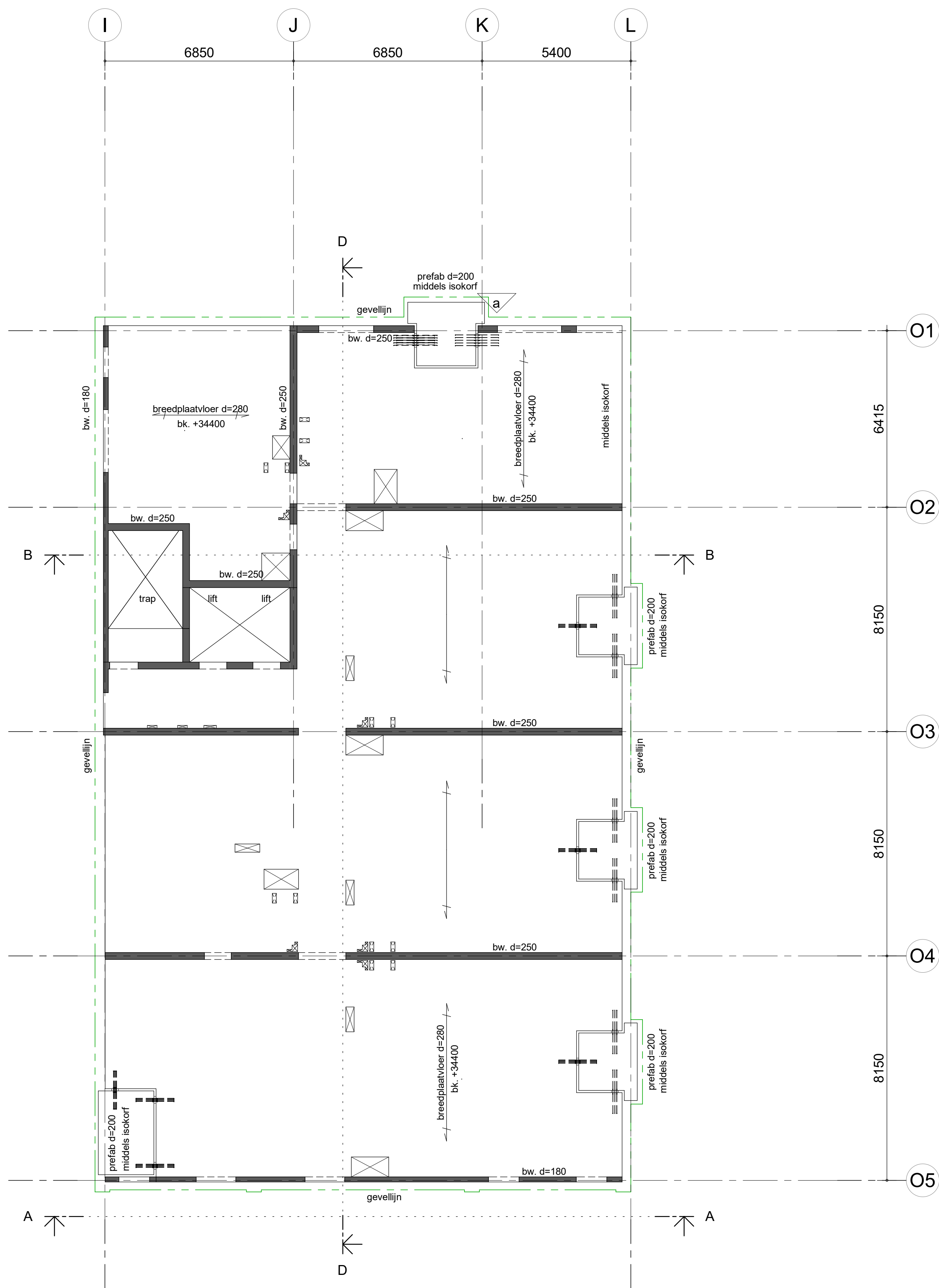
plattegrond 11e verdieping 1 : 100
