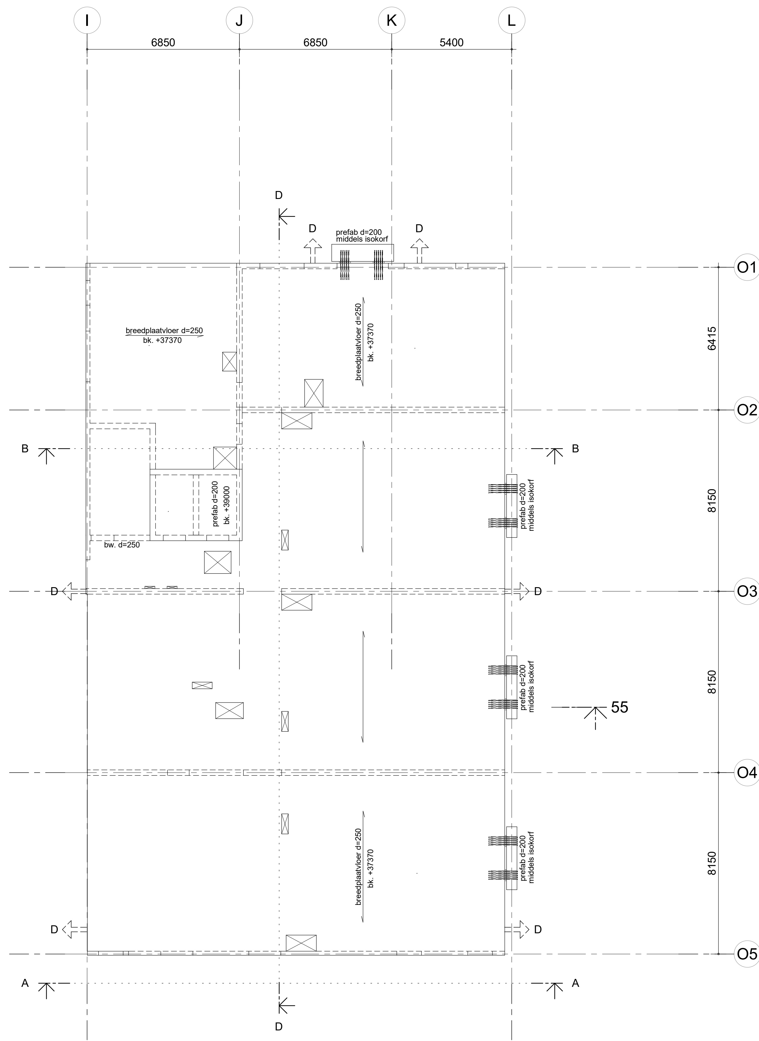
plattegrond Dakvloer 1 : 100
