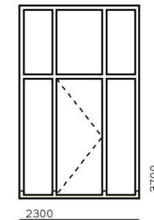
MERK-4 HARDHOUTEN ENTREEKOZIJN MET DTS ONDERDORPEL
