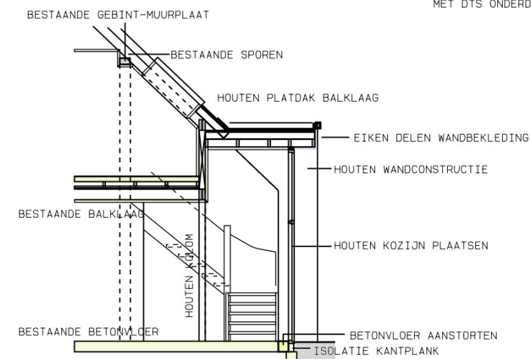
DOORSNEDE
