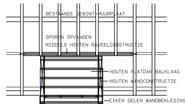
KAPCONSTRUCTIE
