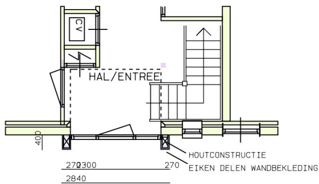
PLATTEGROND
