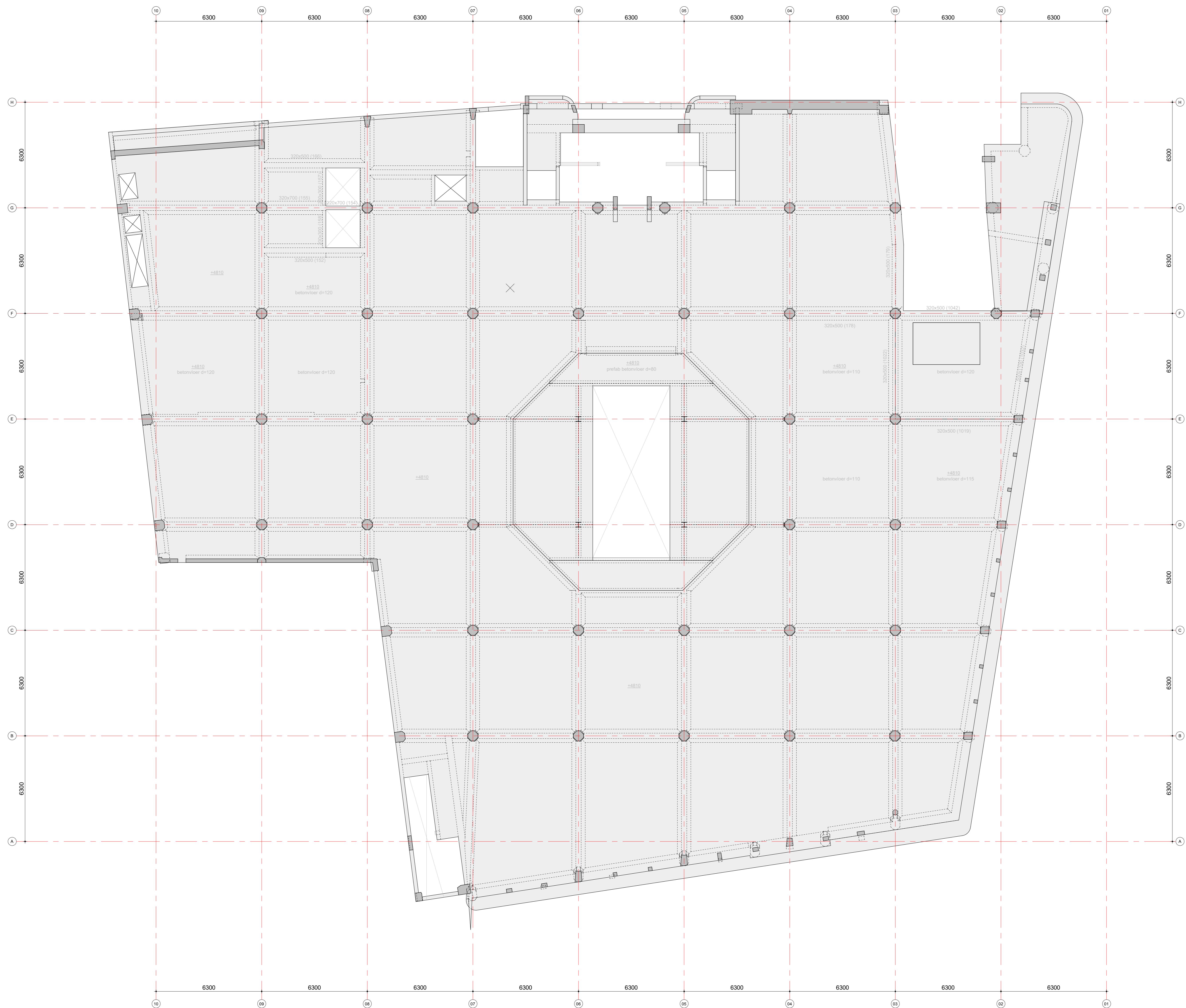
01 eerste verdieping (HS)
