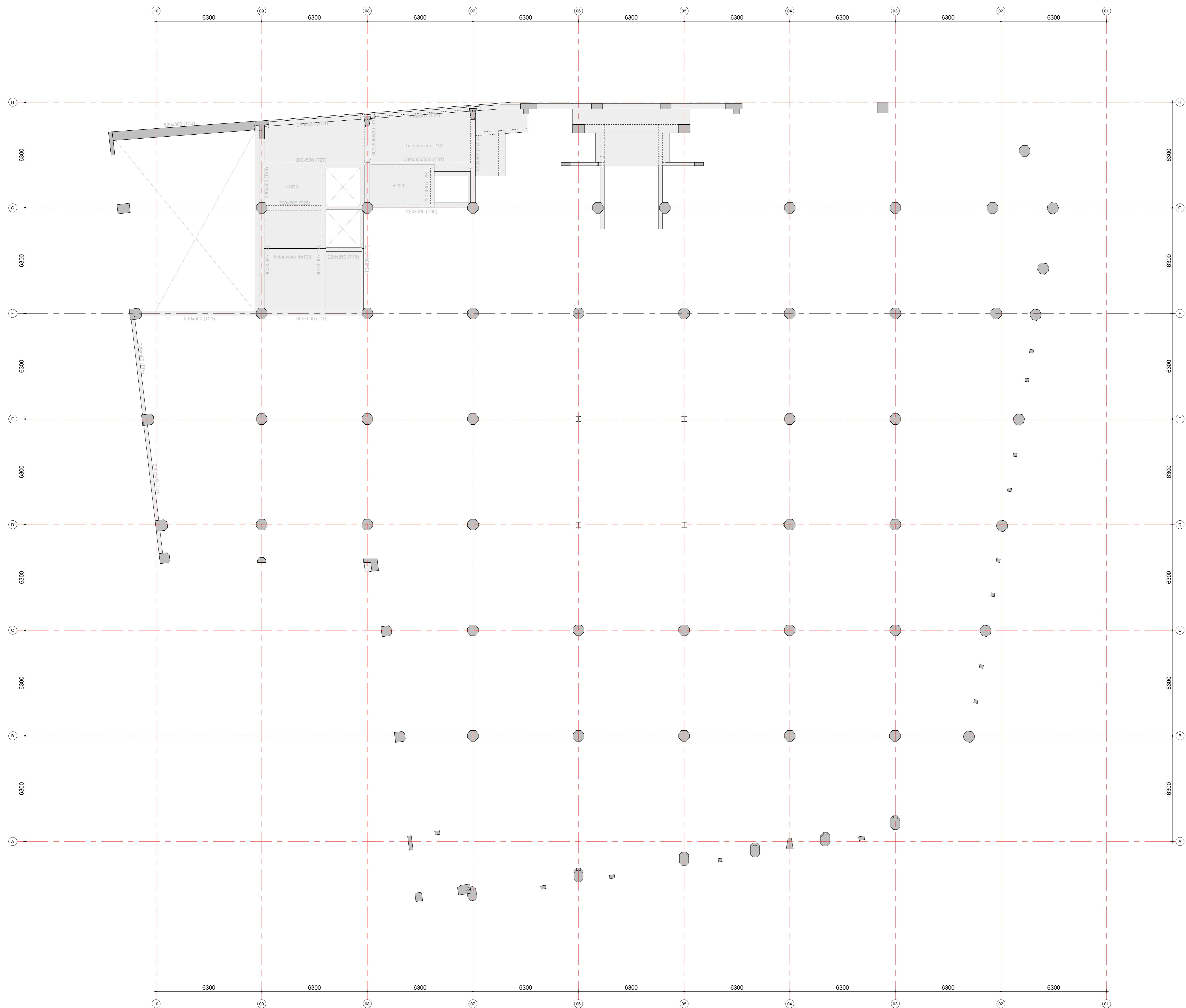
00a tussenverdieping (HS)
