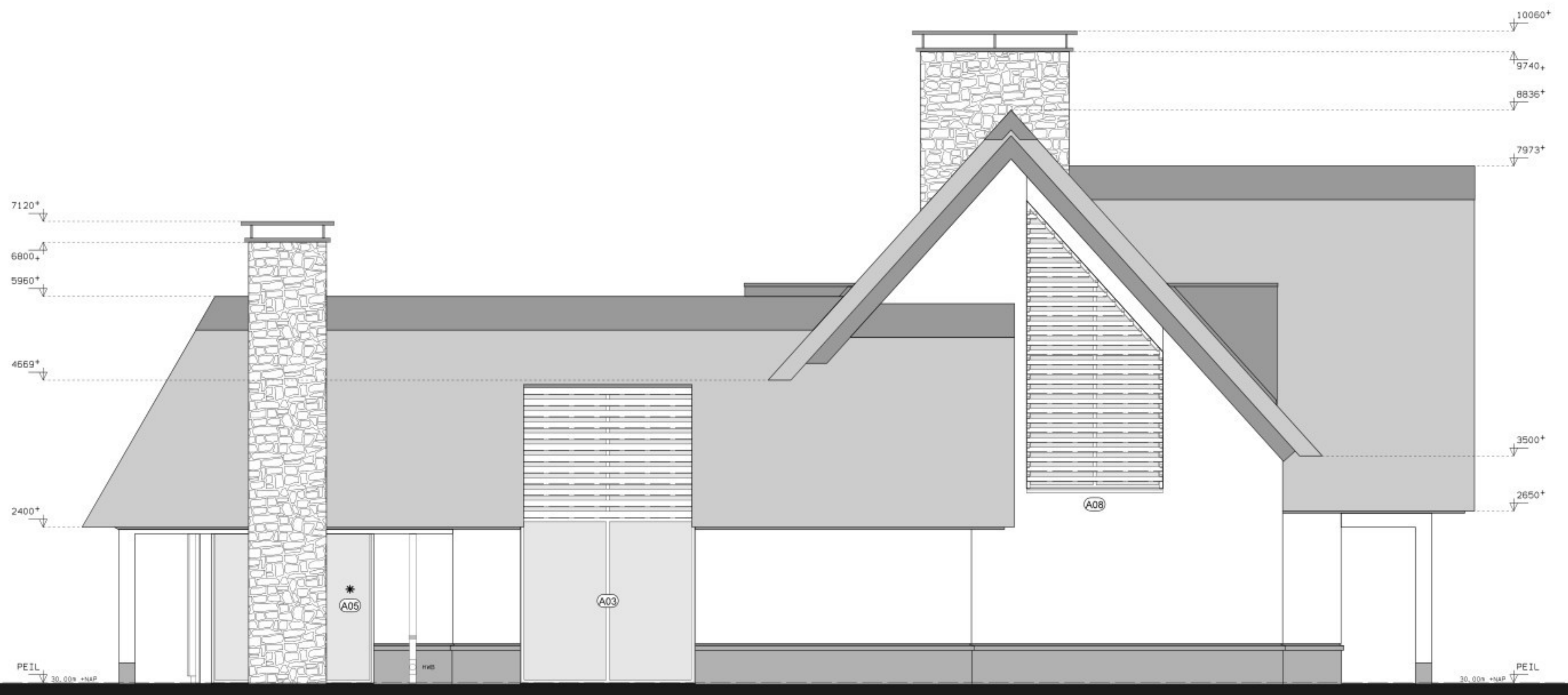
Gevel links
