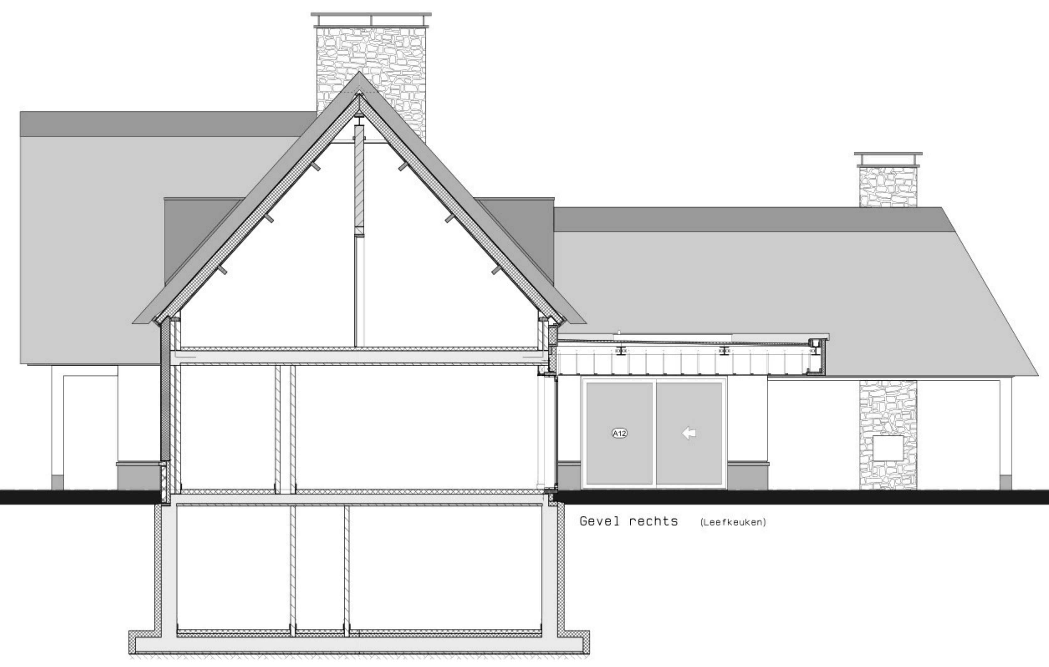
Gevel rechts
