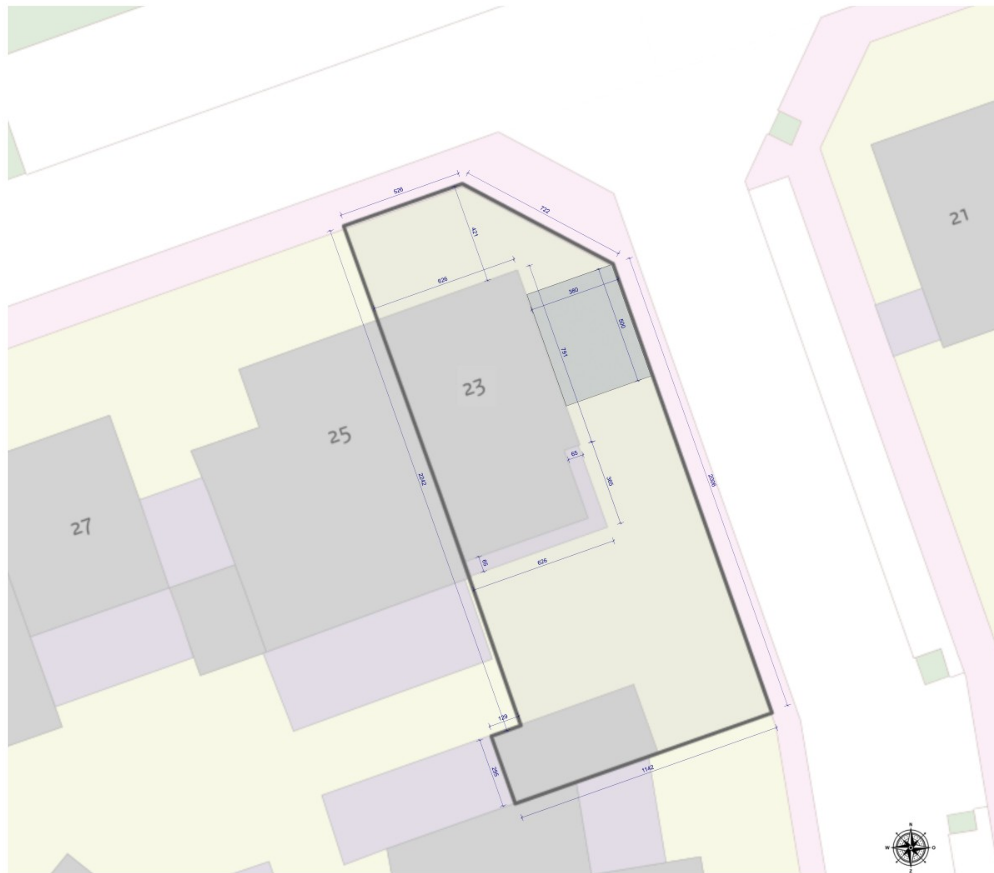
Bovenaanzicht
