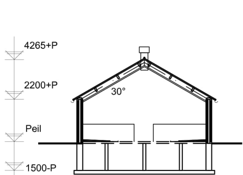
Doorsnede A-A gebouw: 1
