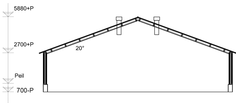
Doorsnede B-B gebouw: 3
