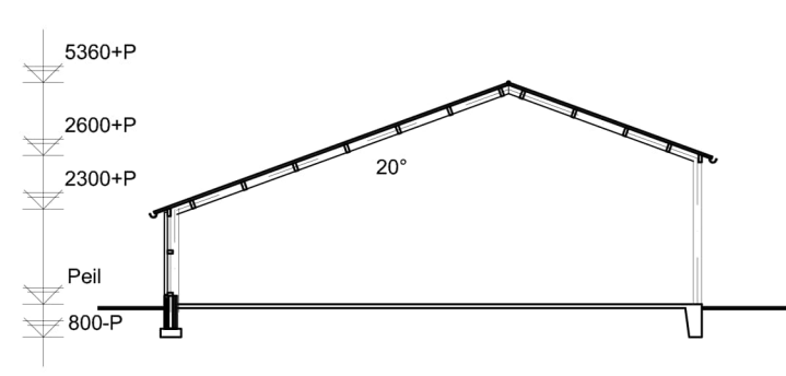
Doorsnede C-C gebouw: 4
