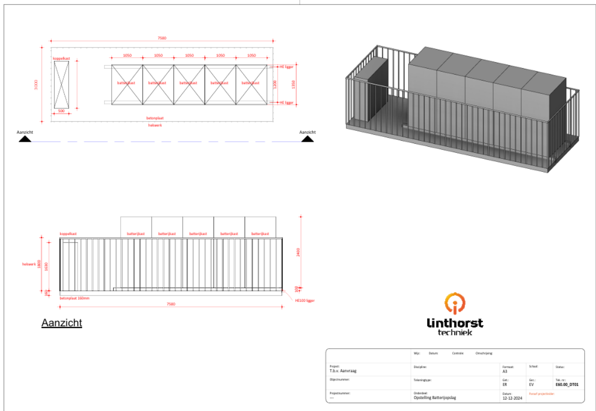
Figuur 2: Weergave van de batterij-opstelling.
