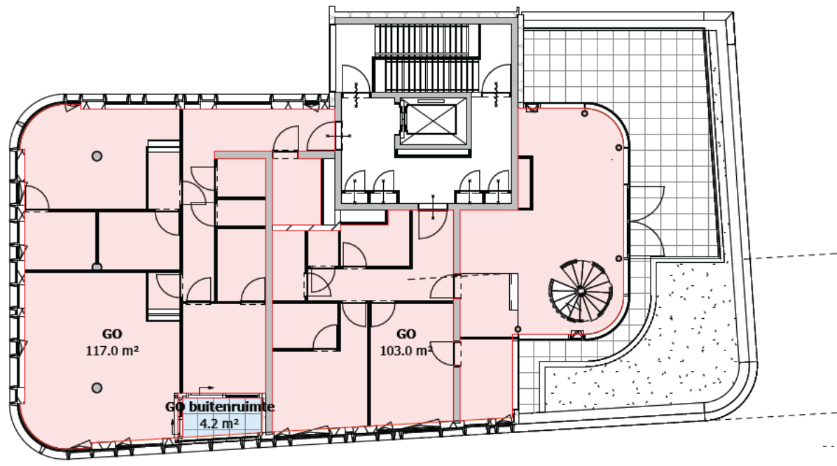
6 4.1 Verdieping schaal 1 : 200
