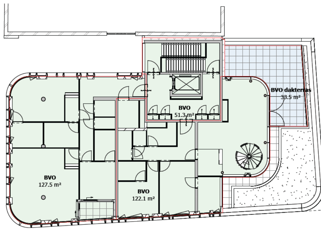
6 4.1 Verdieping
