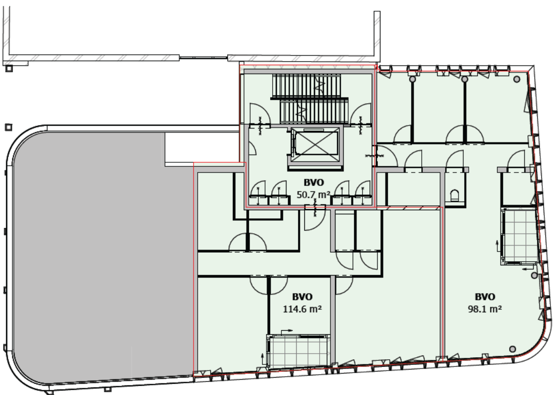
3 1e Verdieping
