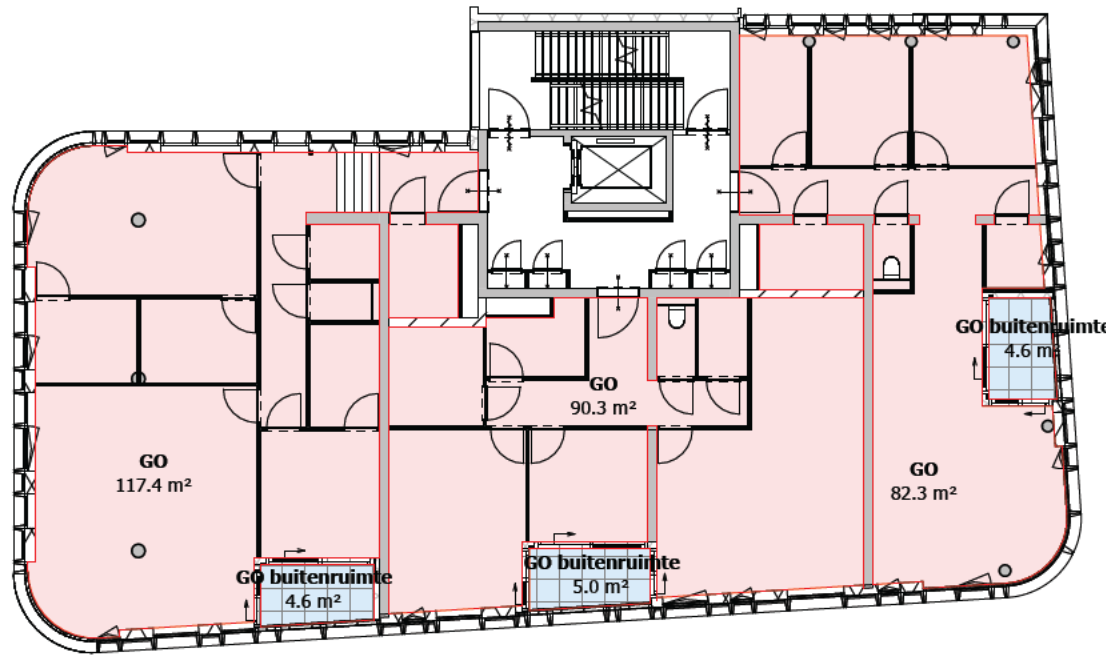
5 3.1 Verdieping schaal 1 : 200
