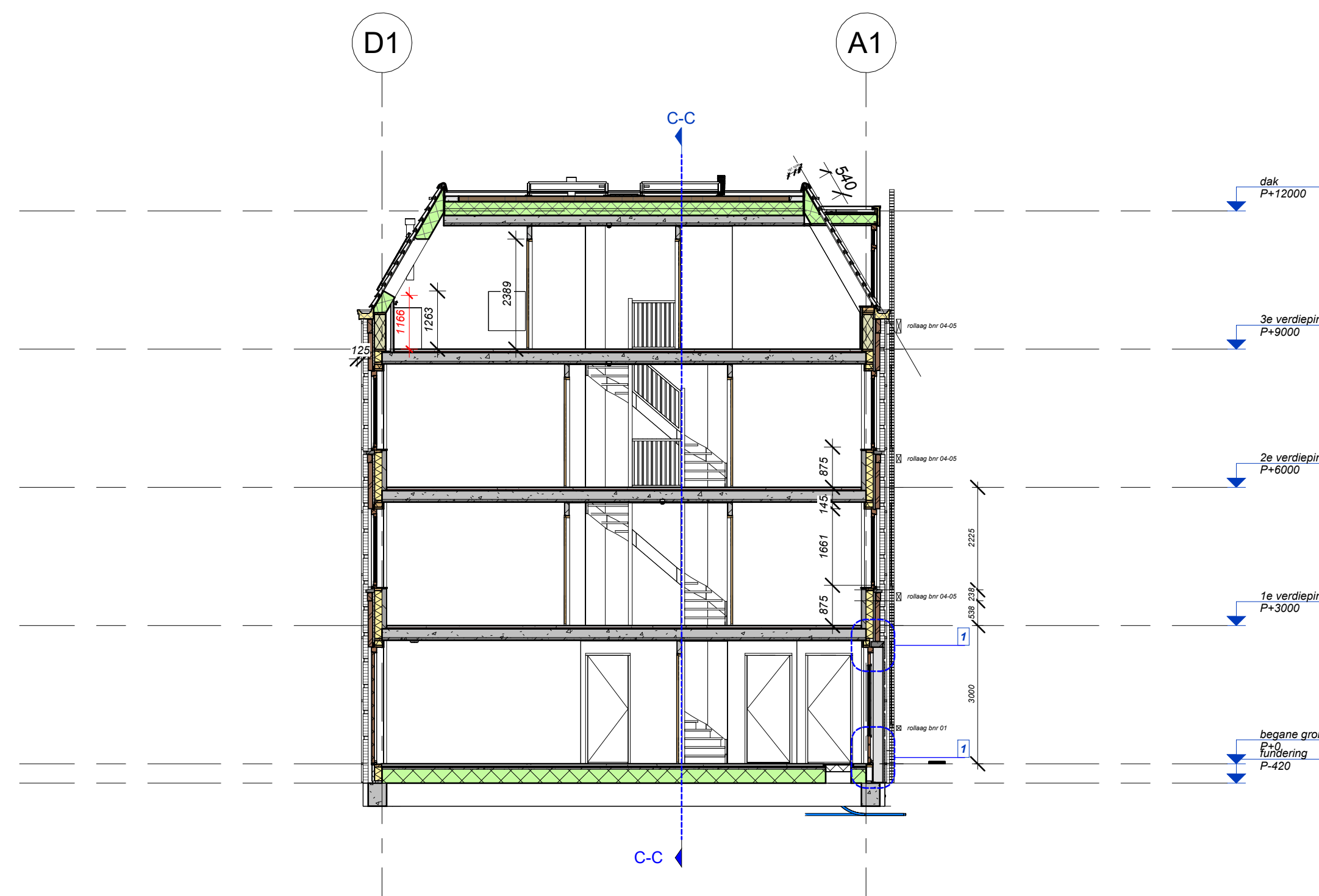
MBB E-E 1 : 100
