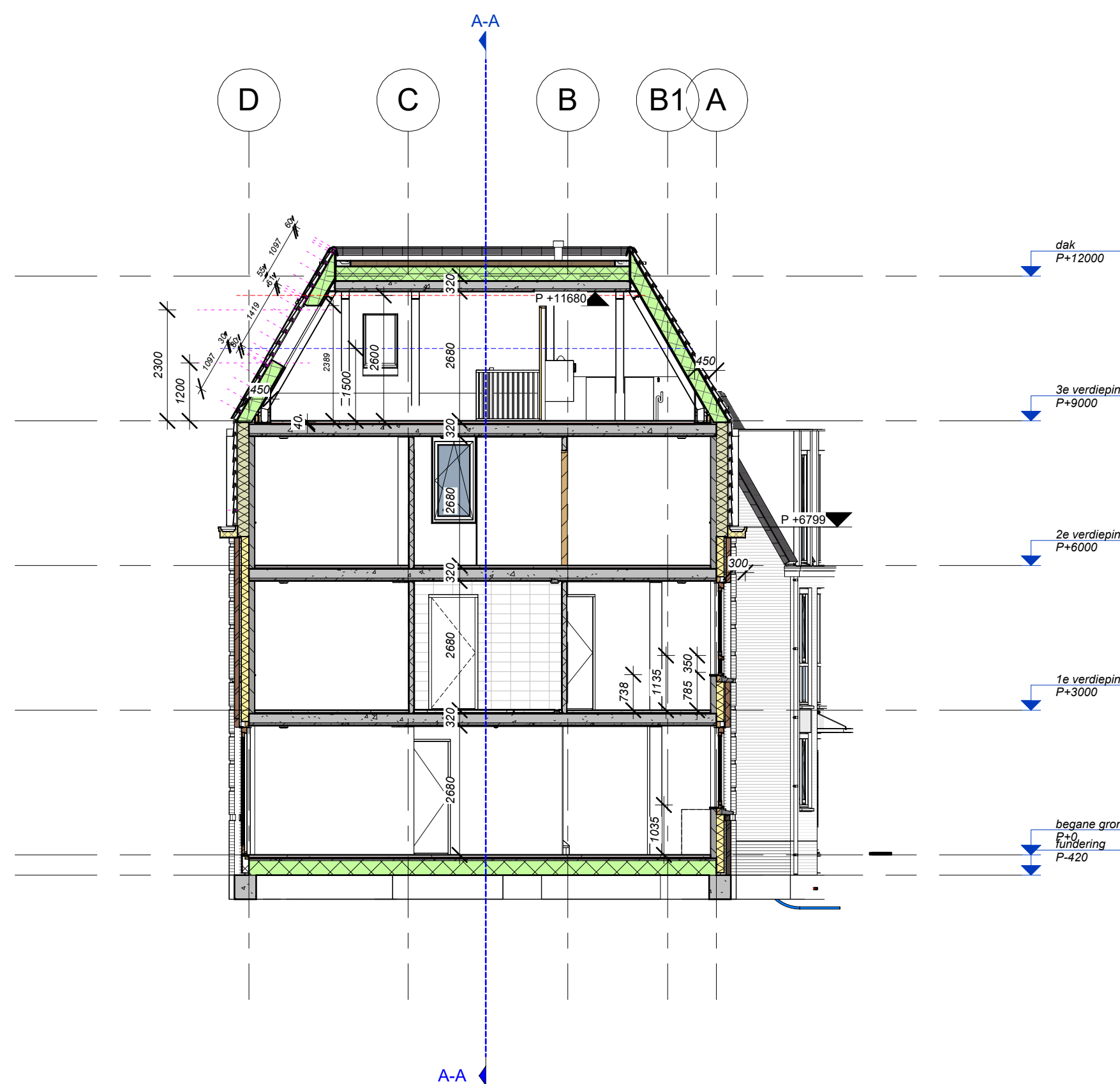
MBB B-B 1 : 100
