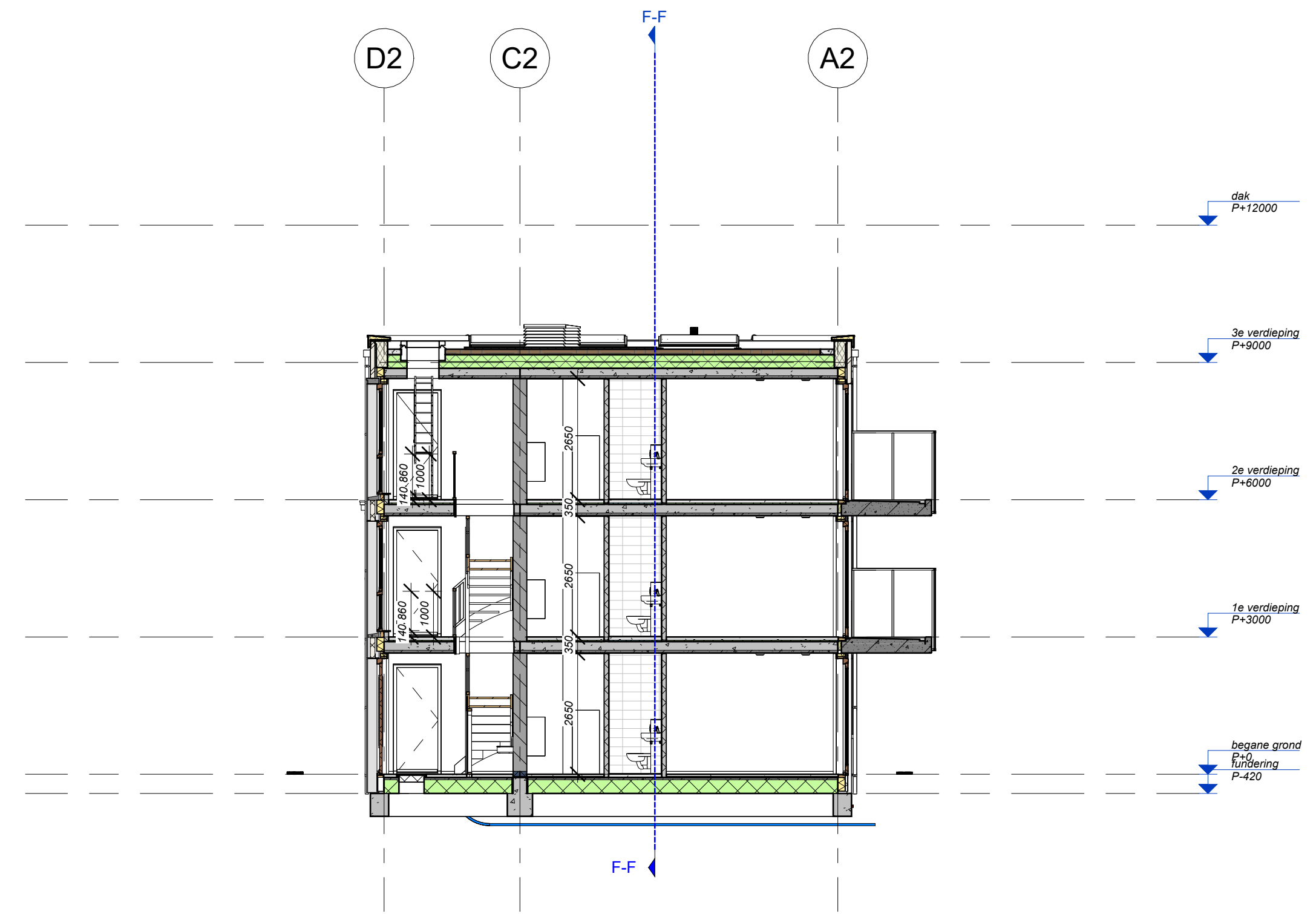
MBB G-G 1 : 100
