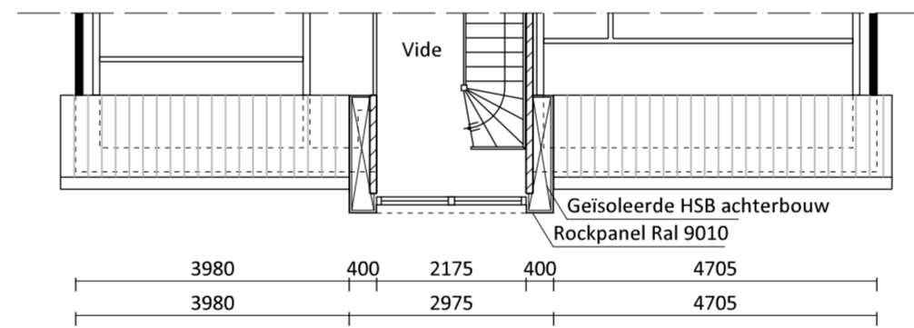
1e Verdieping
