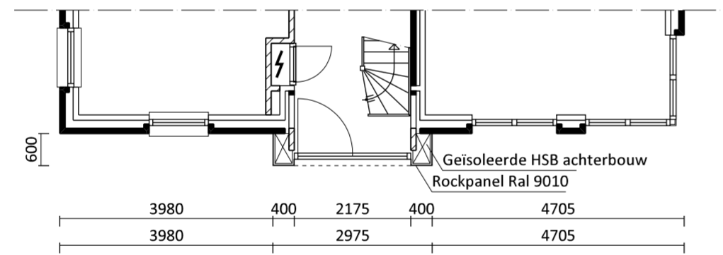
Begane Grond
