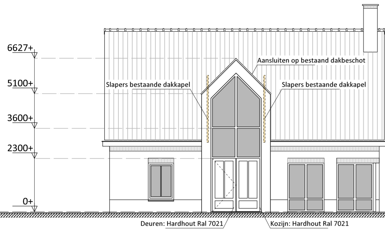
Vooraanzicht
