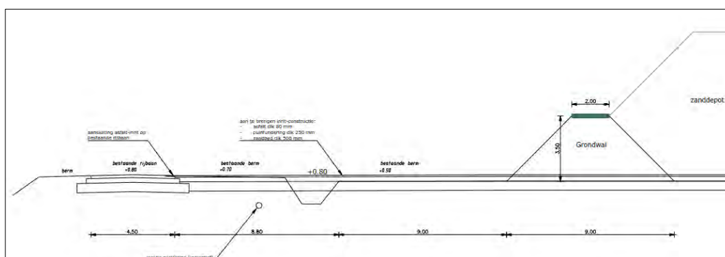
Figuur 5.3 Doorsnede B-B
