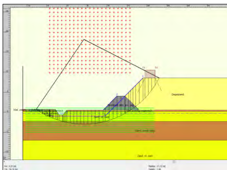
Figuur 5.6 Afschuifcirkel door of onder de gasleiding door ( F_{min} \geq 1,38 ).
