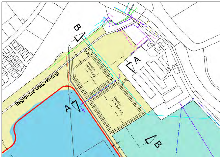
Figuur 2.3 Detailtekening toekomstig zanddepot
