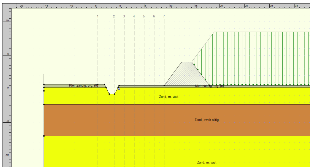
Figuur 5.8 Dwarsprofiel met rekenverticalen
