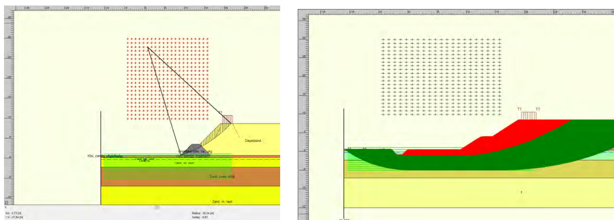
Figuur 5.5 Afschuifvlak met minimale stabiliteitsfactor ( F_{min} = 0,63 )
