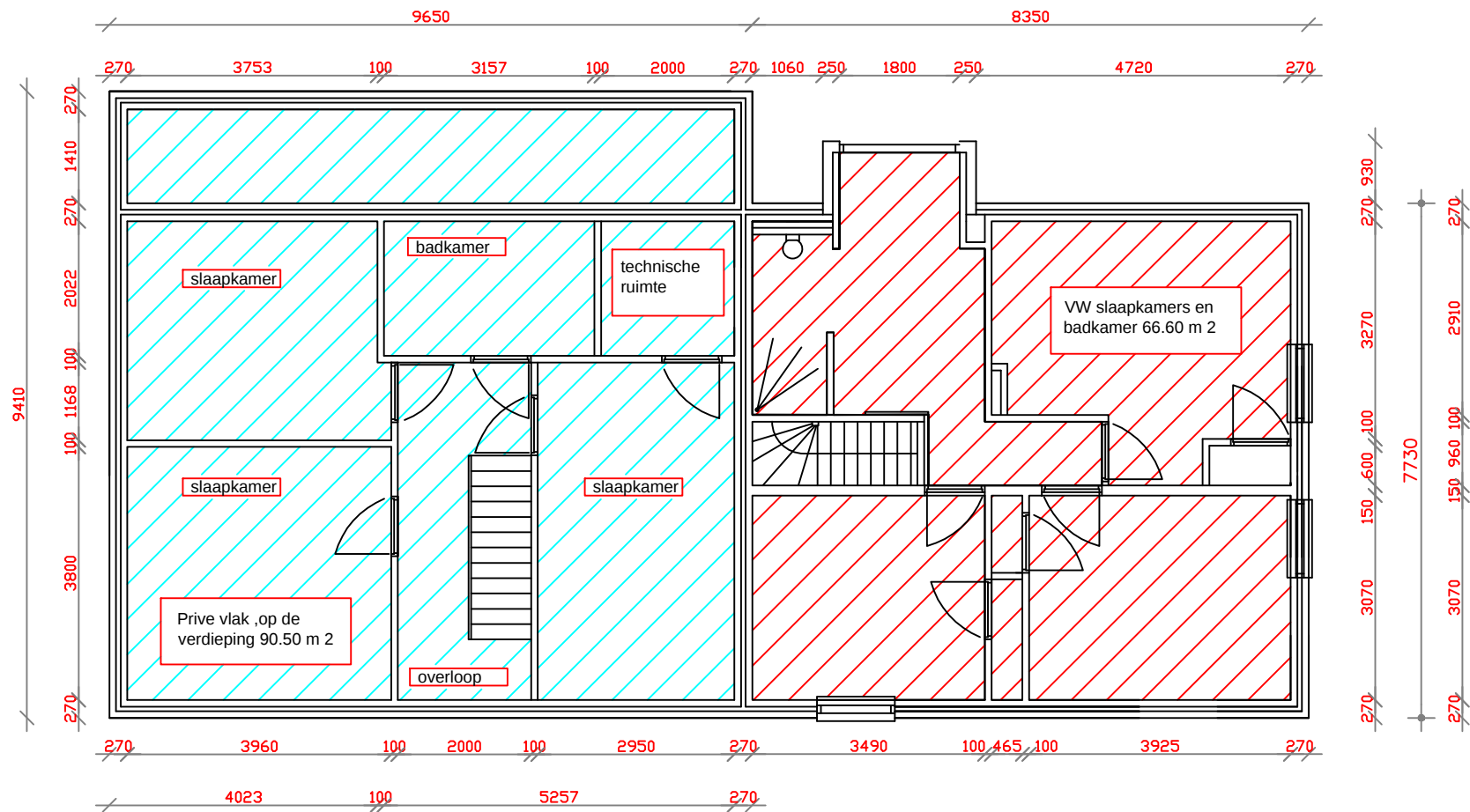
1.e verdieping van woning Toon Kortooms Park Griendtsveenseweg 80 Deurne rode arcering is vakantiewoning en groene arcering is prive.
