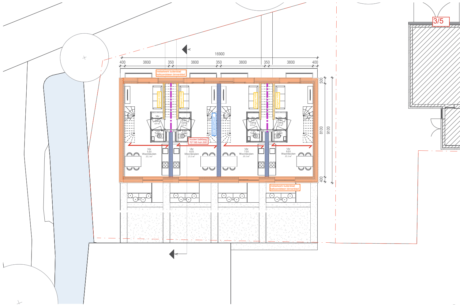
Plattegrond 1ste verdieping
