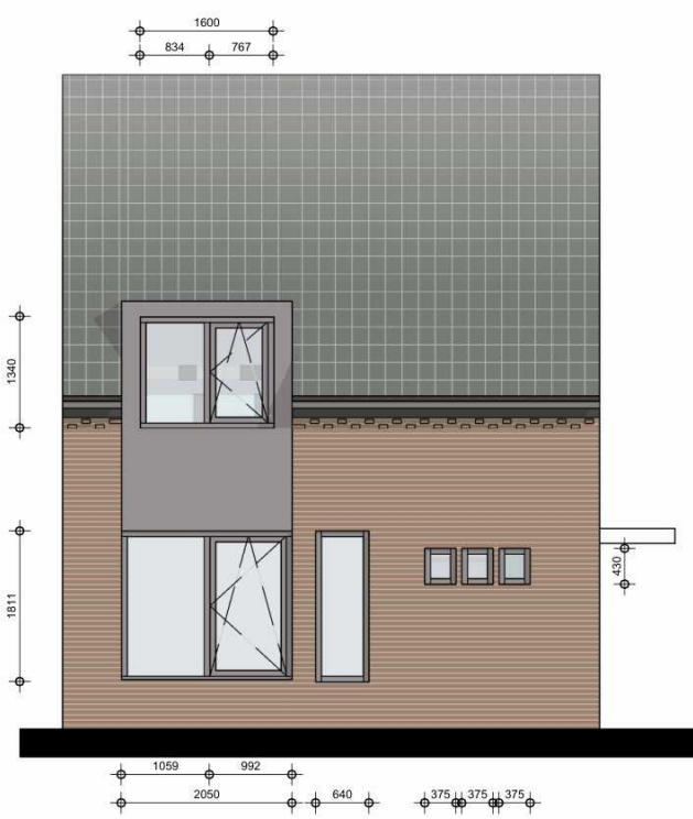
Voorgevel hoekwoning
