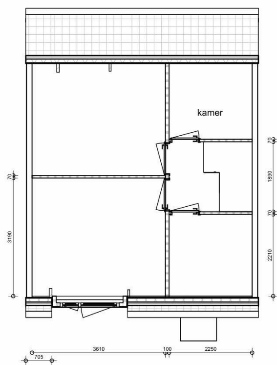
eerste verdieping
