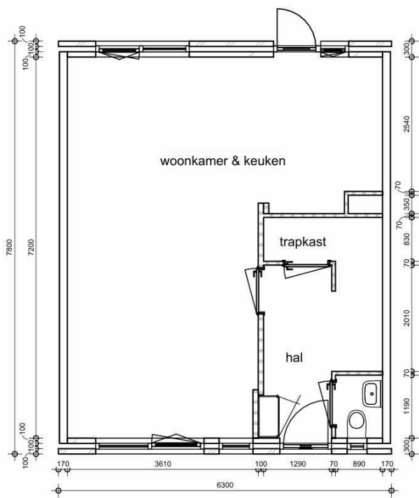
begane grond
