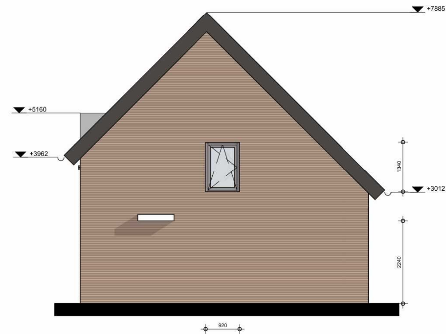
Zijgevel
