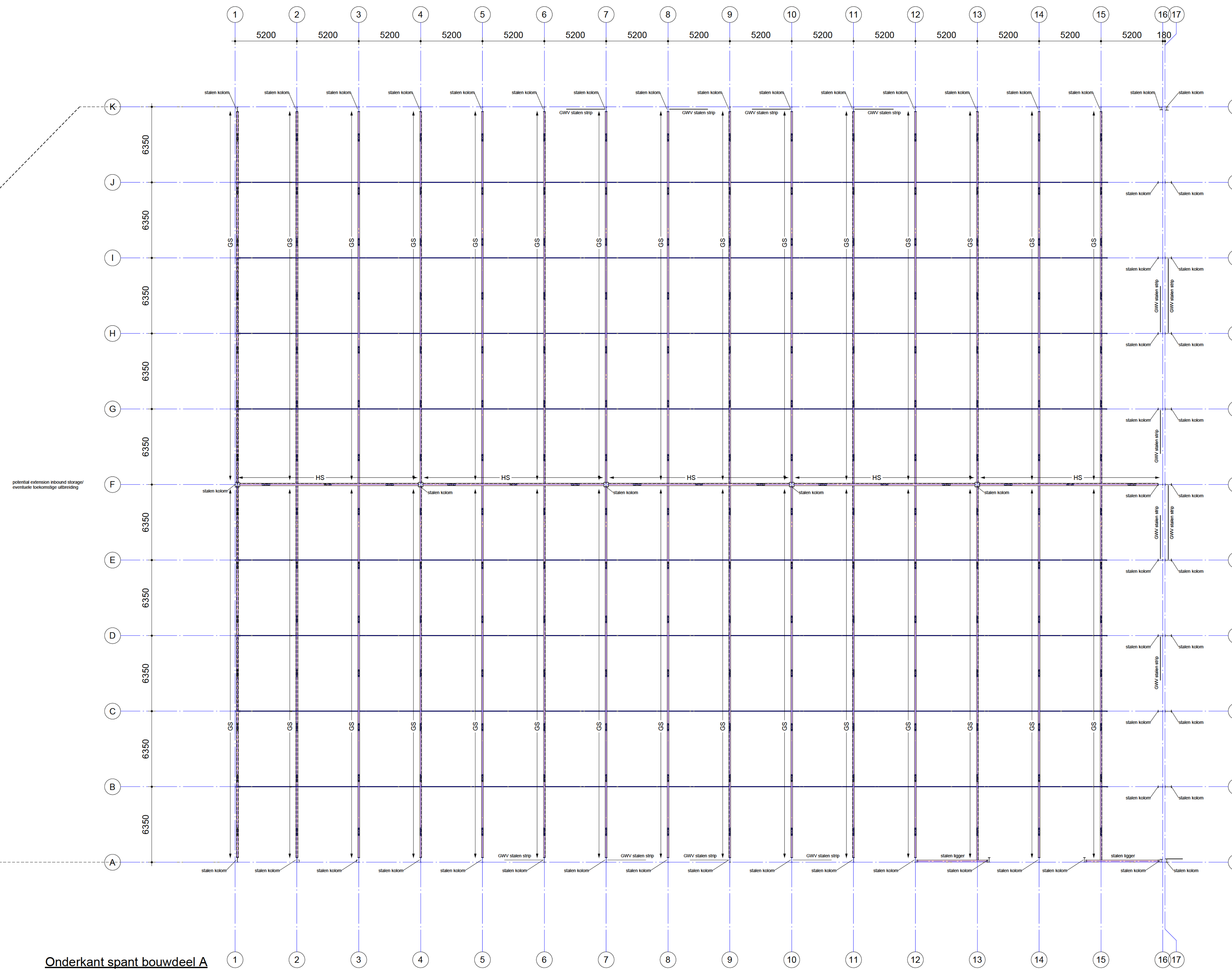
Onderkant spant bouwdeel A
