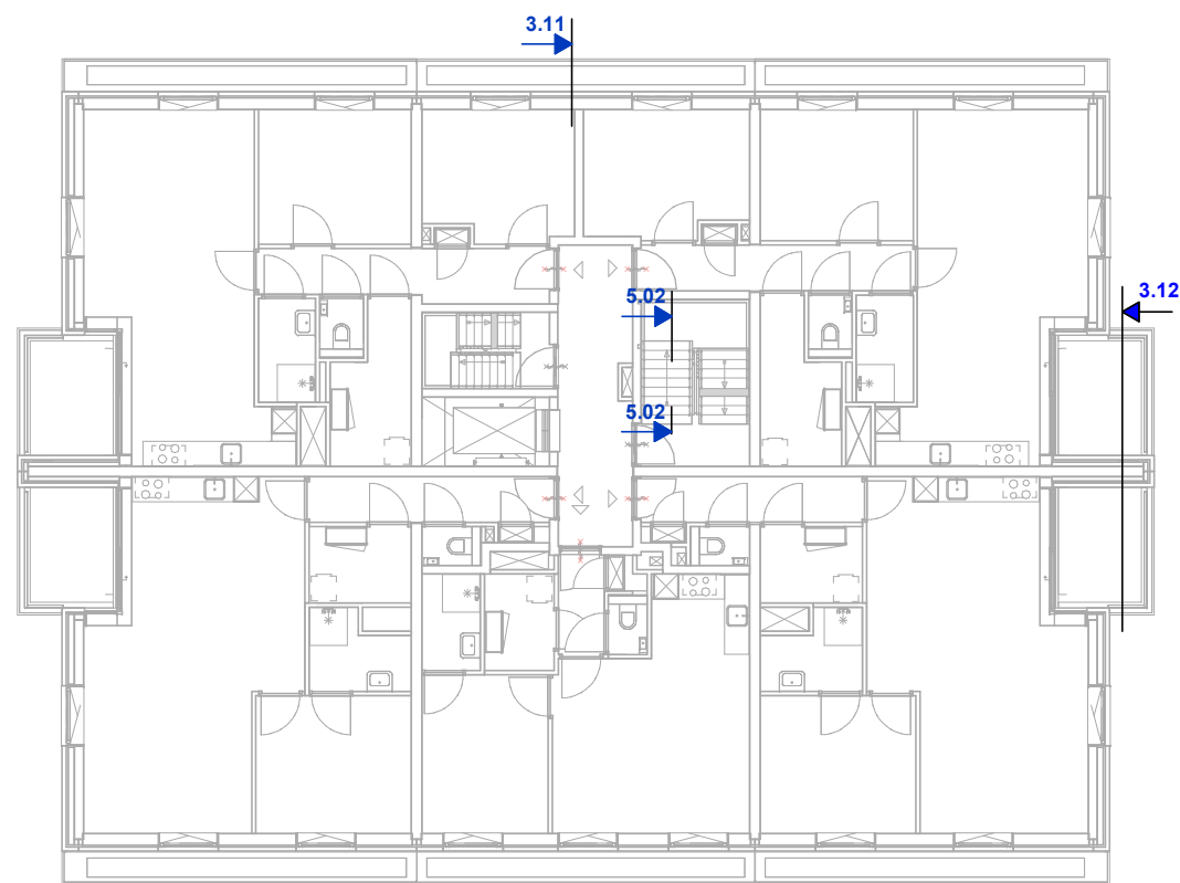
Tweede verdieping
