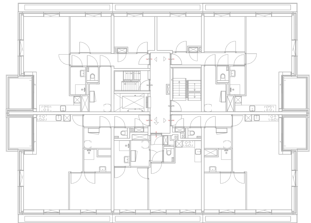
Derde verdieping
