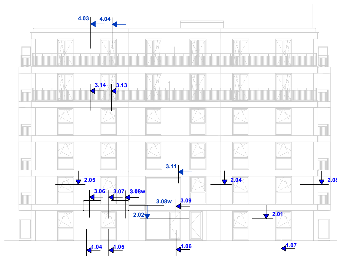
detailoverzicht noordgevel
