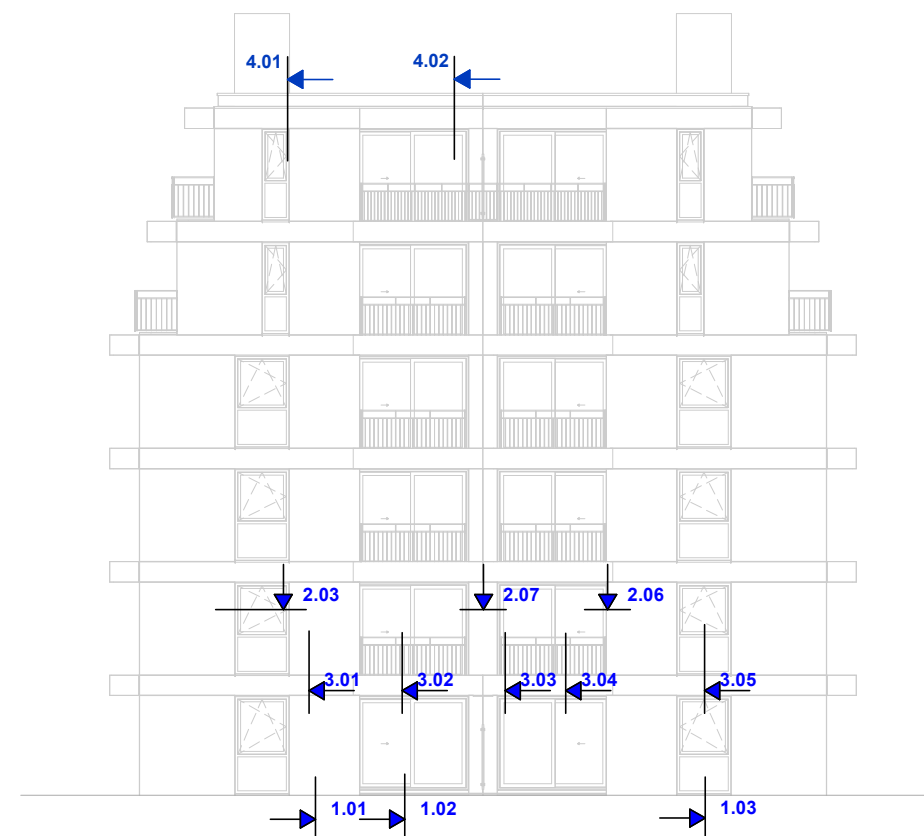
detailoverzicht oostgevel
