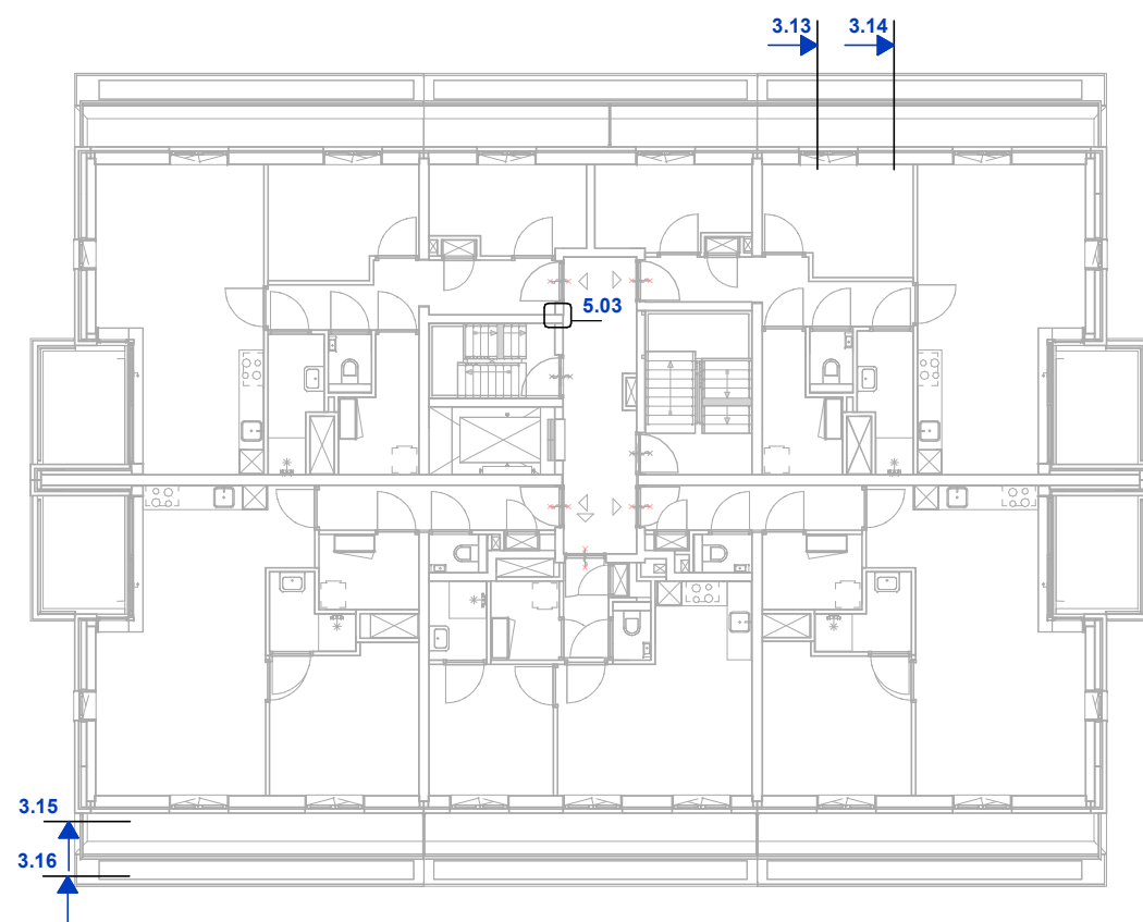
Vierde verdieping
