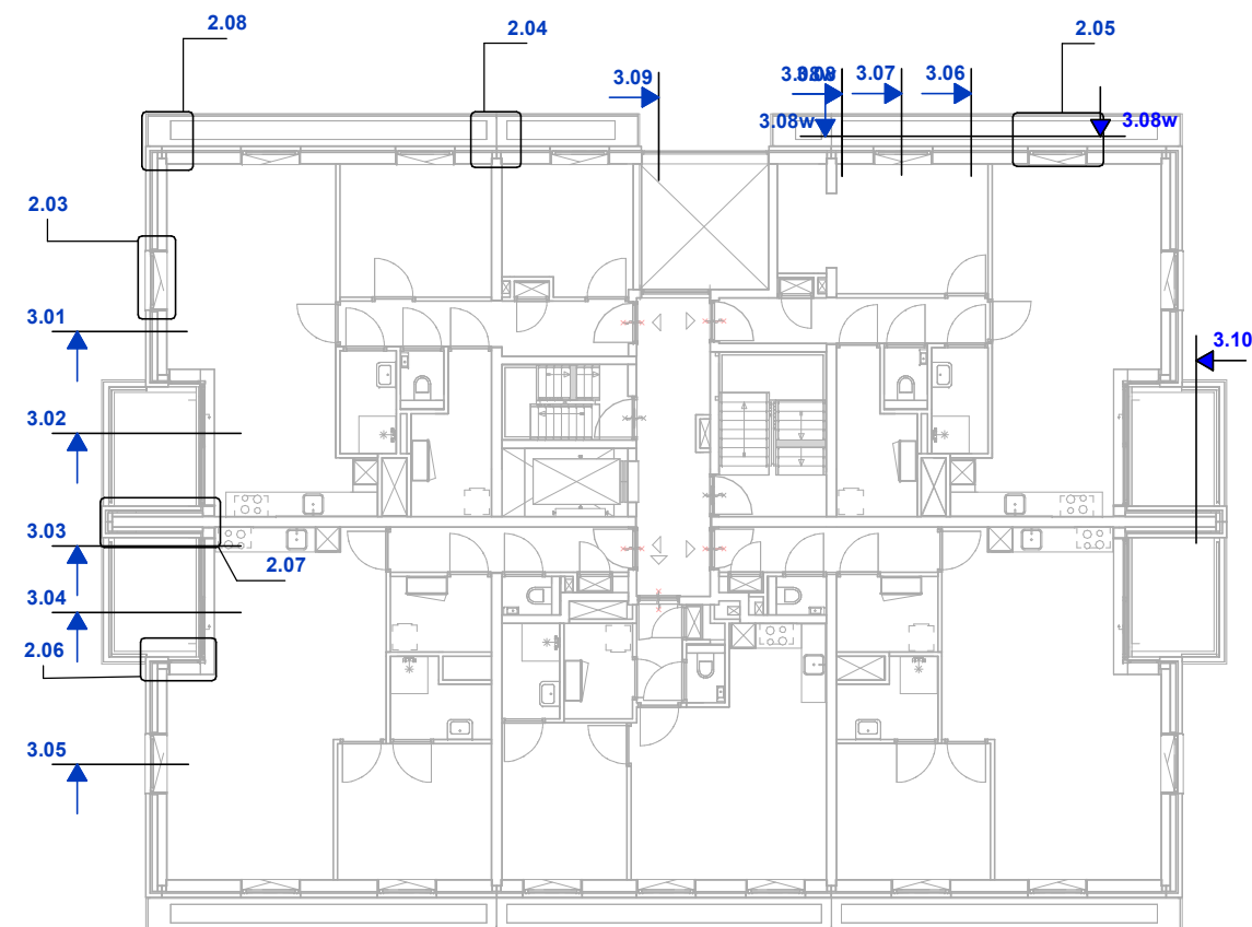
Eerste verdieping
