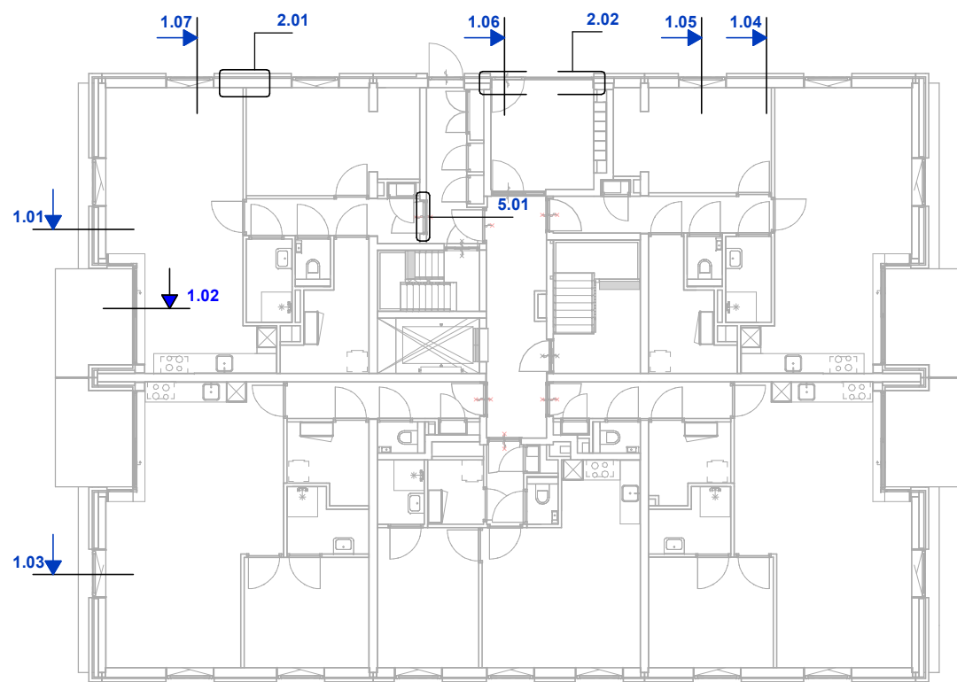
Begane grond
