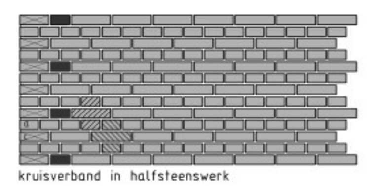
kruisverband in halfsteenswerk
