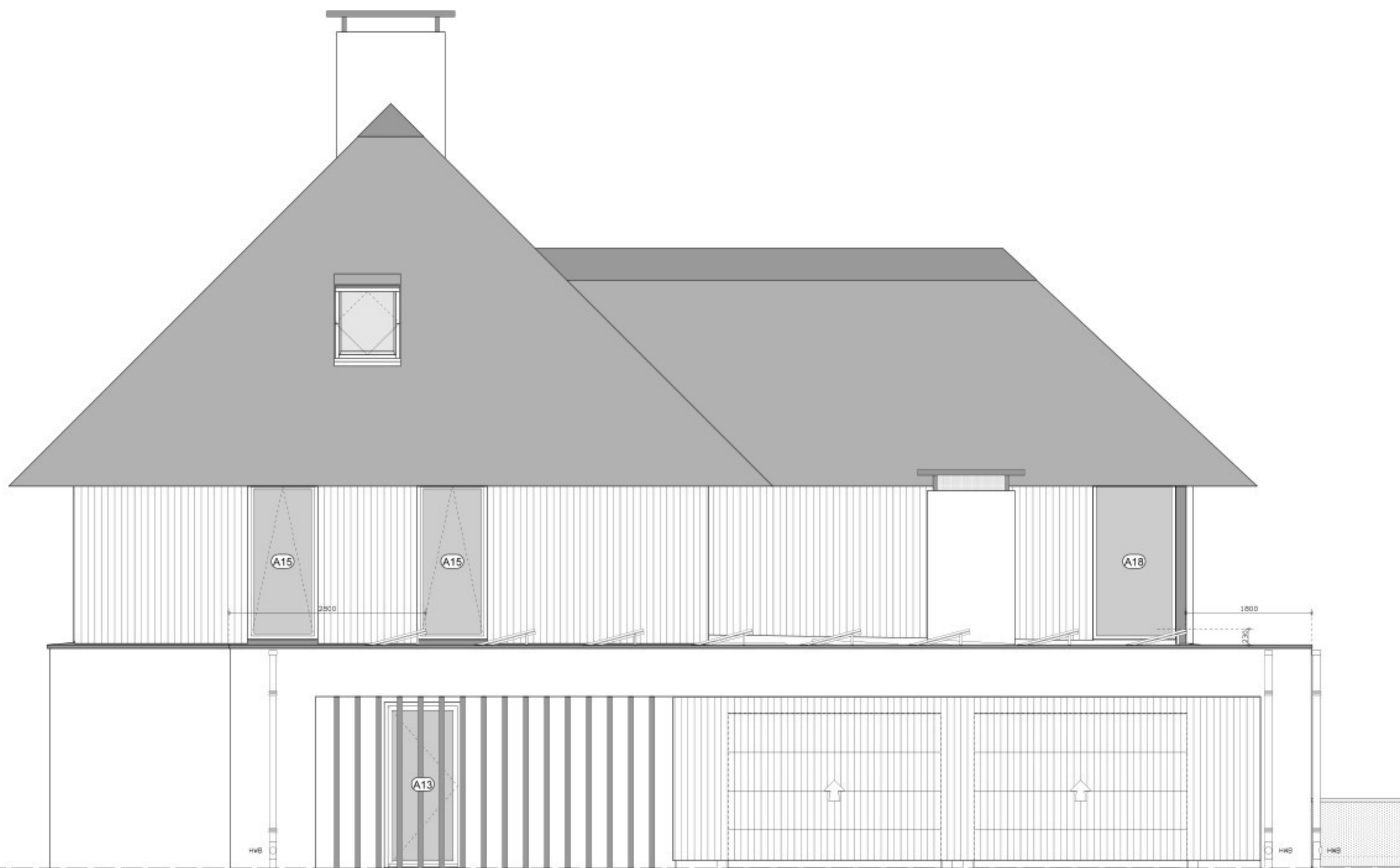
Gevel rechts
