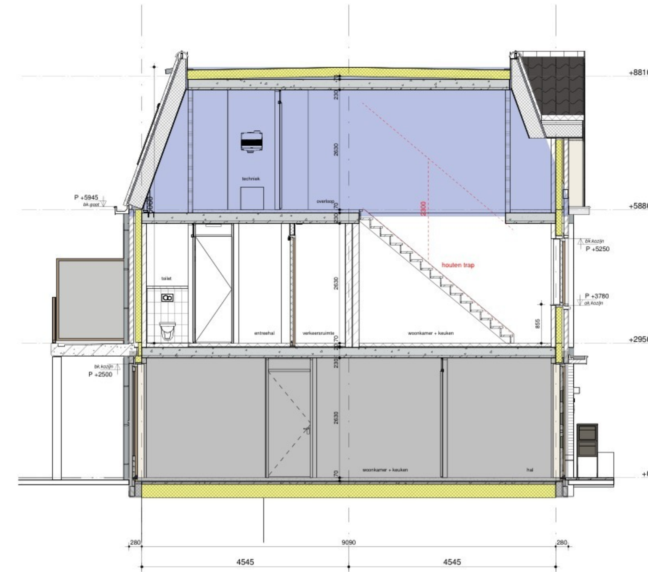
Doorsnede B-B 1 : 50
