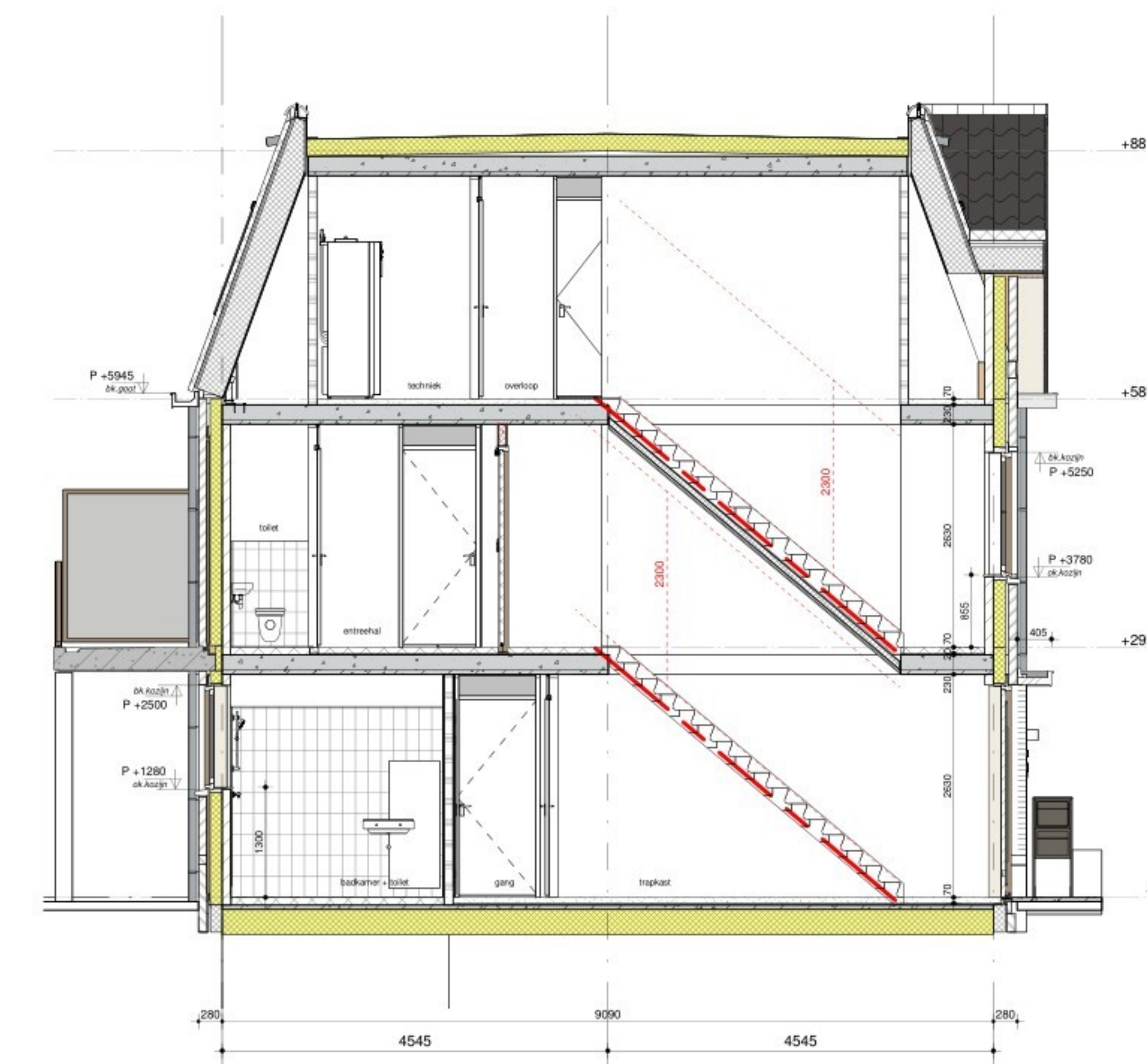
Doorsnede A-A 1 : 50
