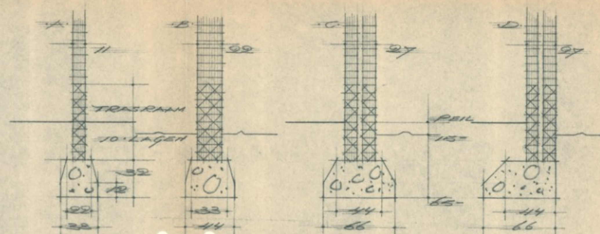
FUNDERINGEN. 1:20.
