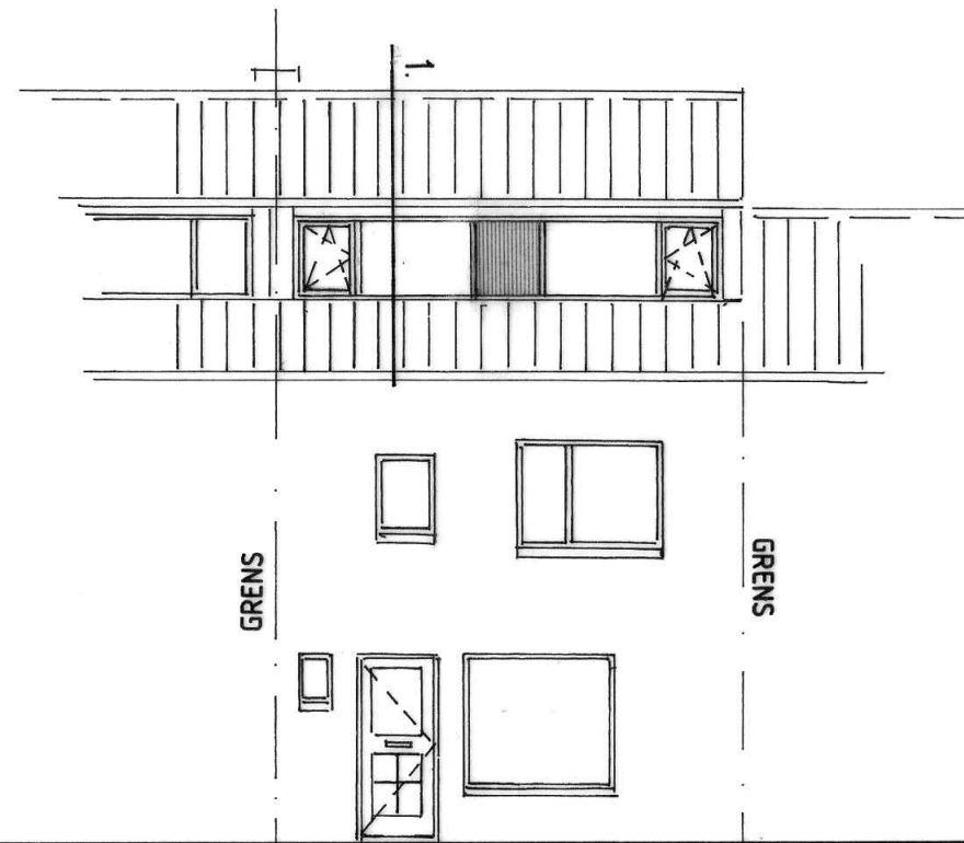
VOORAANZICHT GEWIJZIGD
