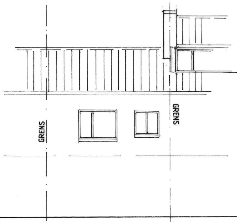
ACHTERAANZICHT BESTAAND
