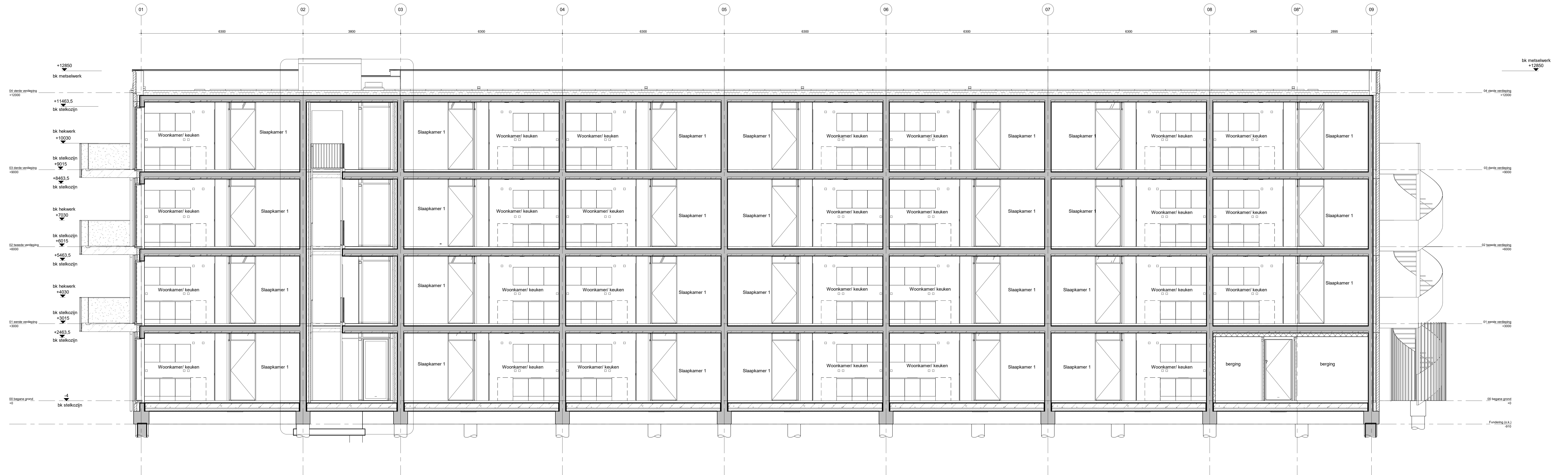
doorsnede tussen as-A en as-B 1:50
