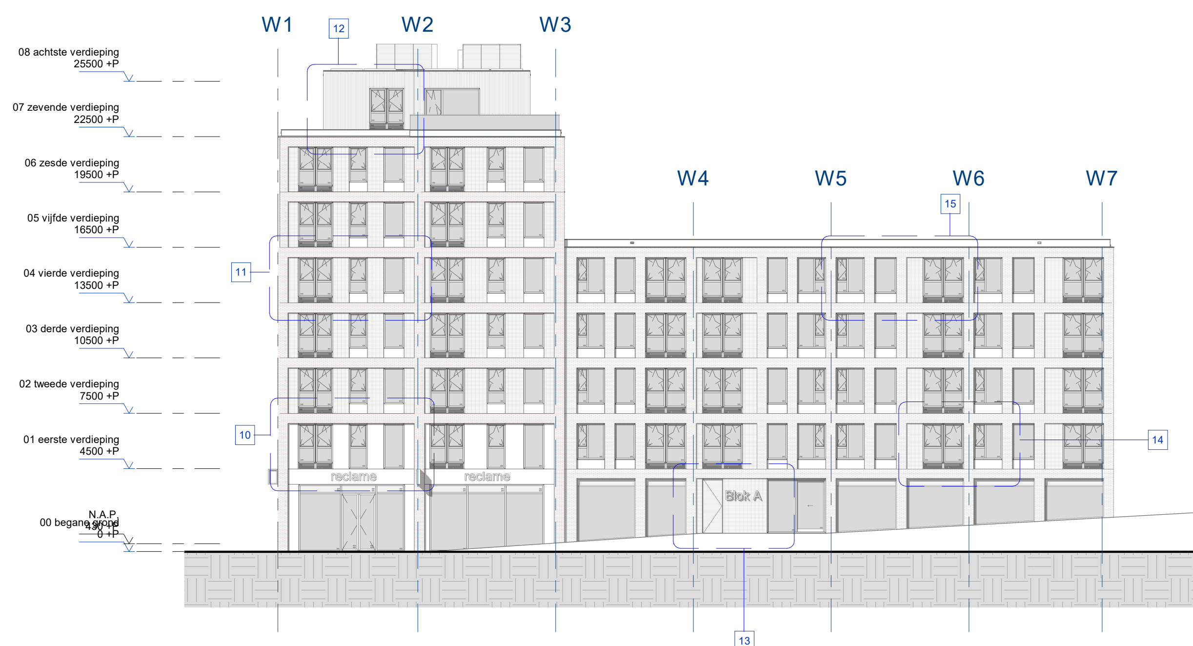
westgevel-fragmenten schaal 1 : 200
