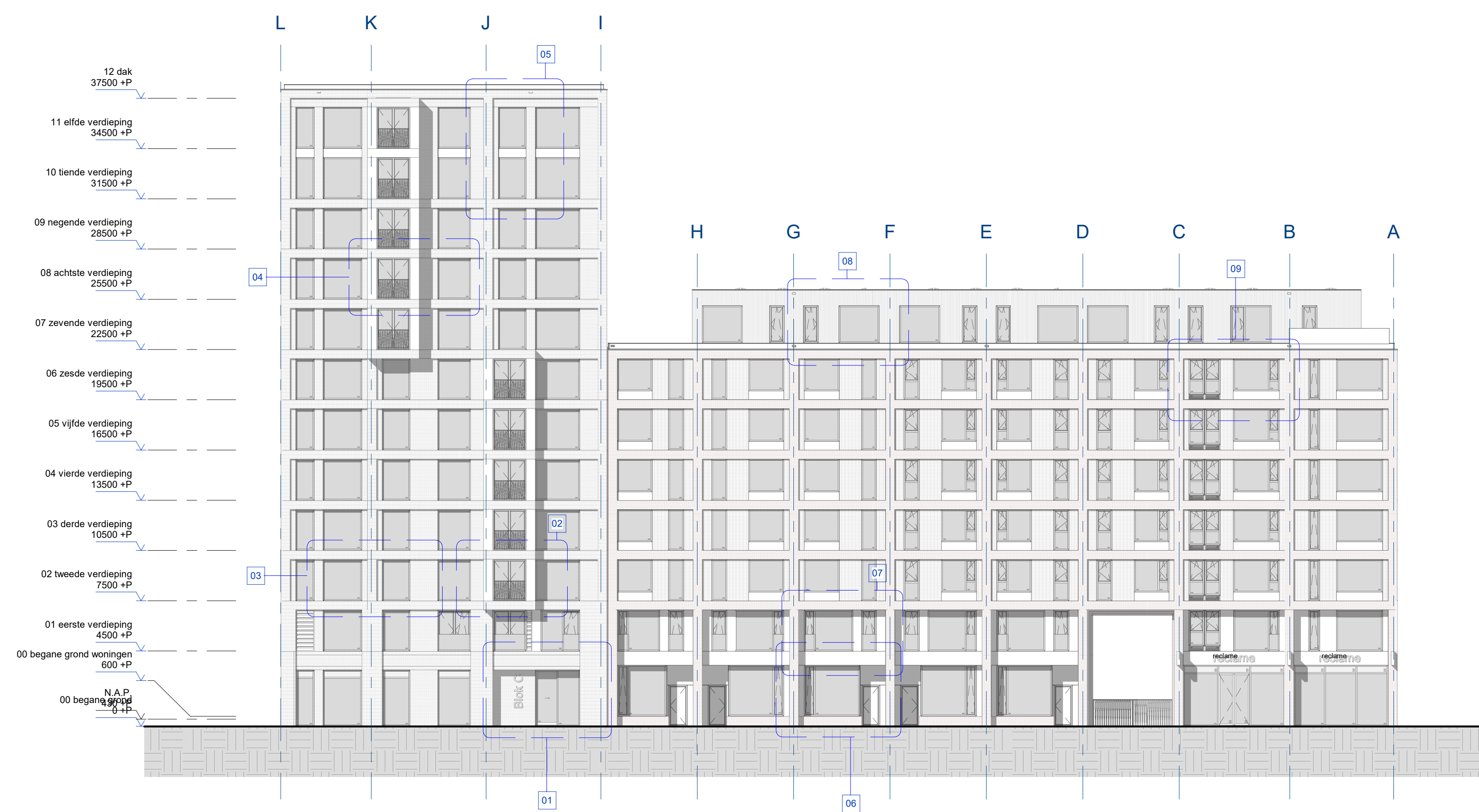
noordgevel-fragmenten schaal 1 : 200
