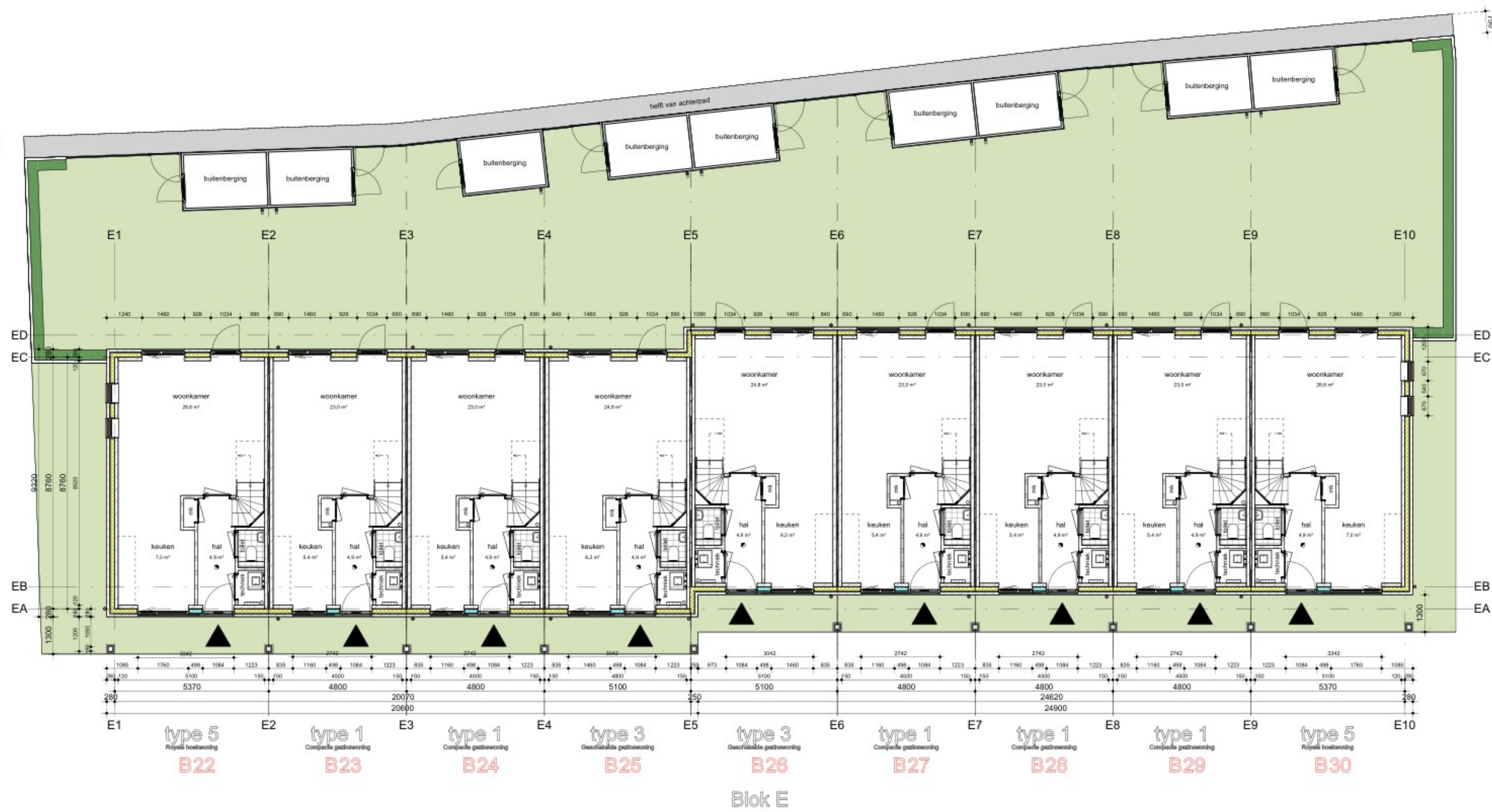
begane grond
