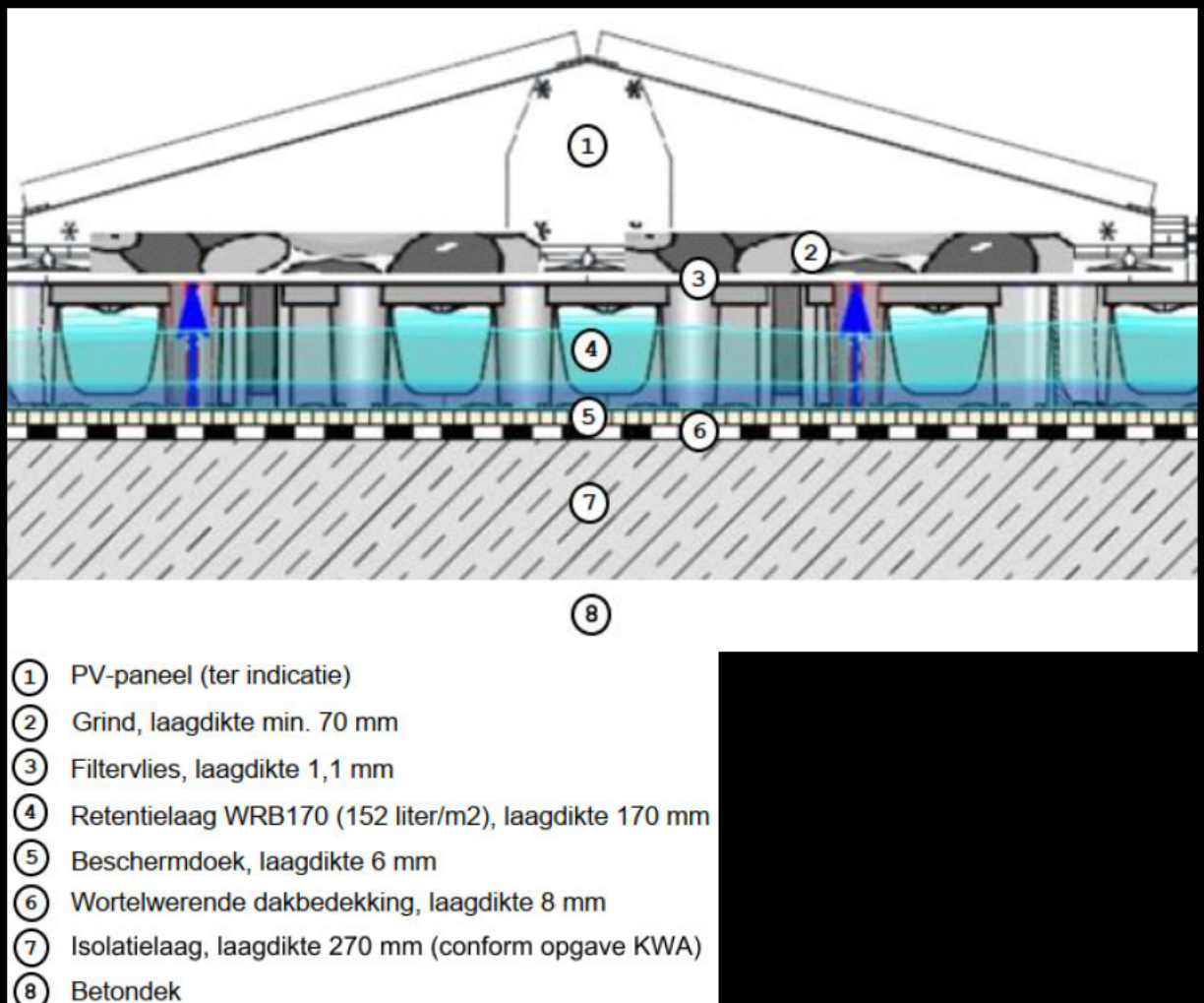
Figuur 12: Principe doorsnede zonnepanelen met grind.
