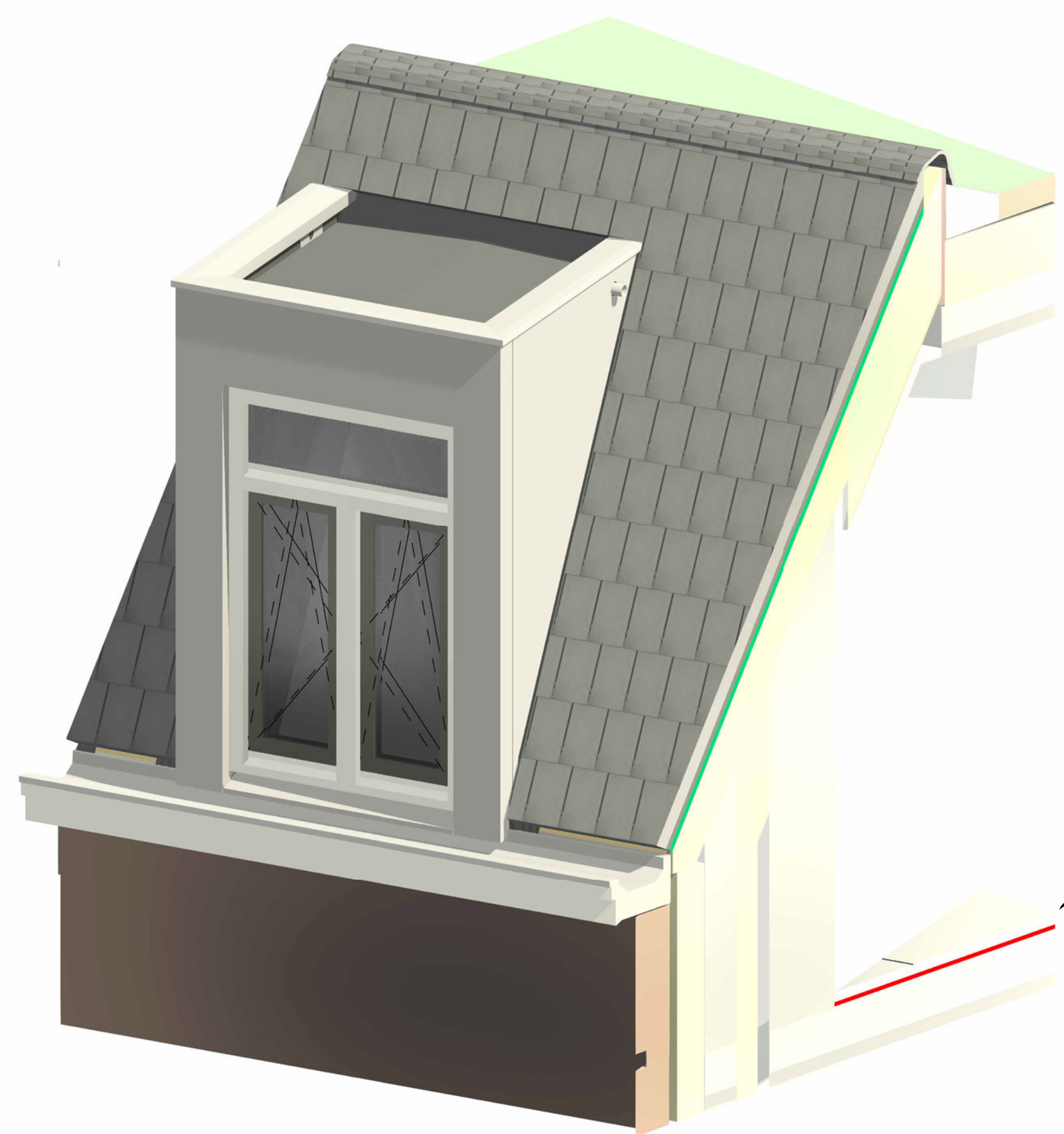
502-A 1 : 20
