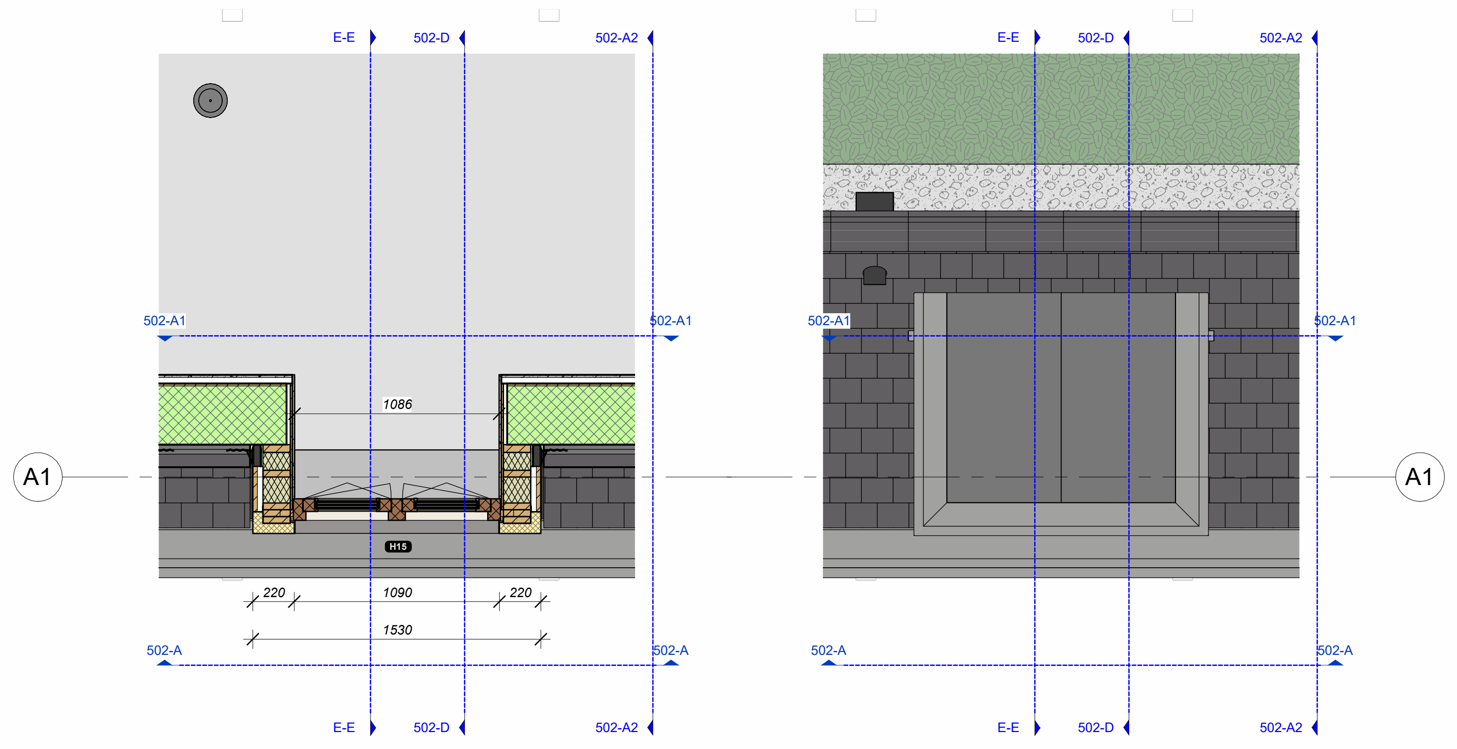
502-P 1 : 20
