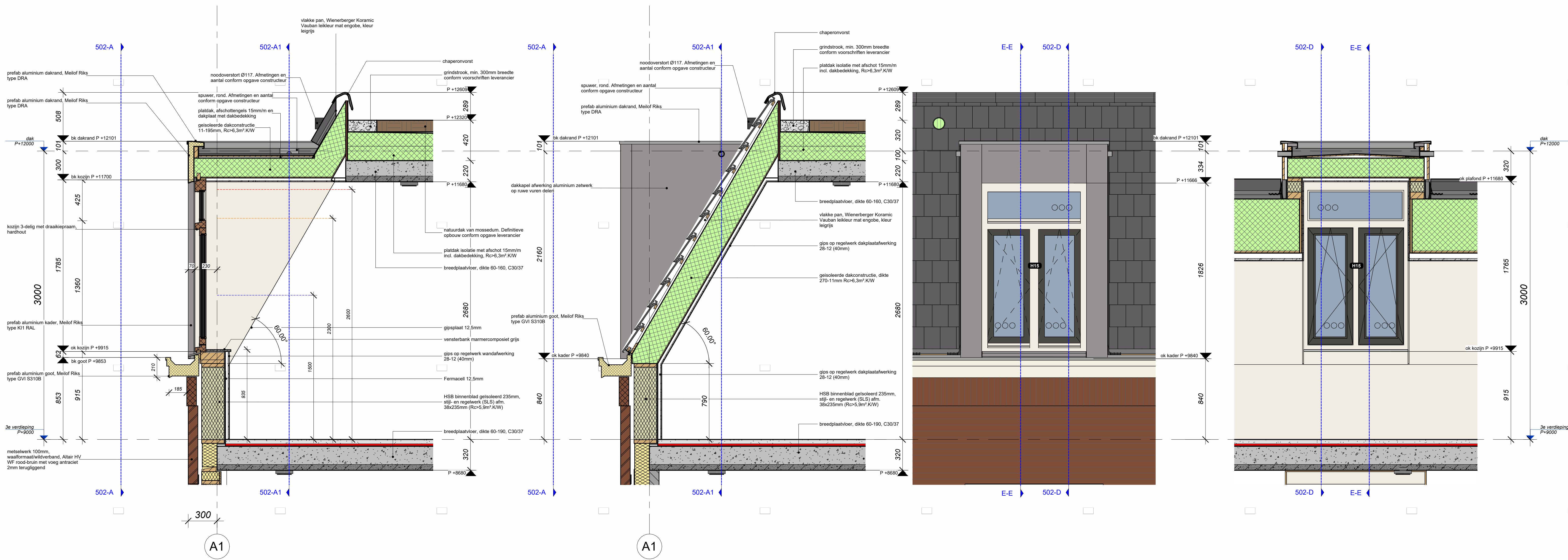
502-D 1 : 20
