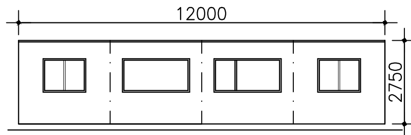
A) Achter aanzicht
