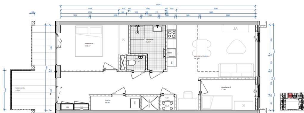
f 5.8 Woningtype B5 (plattegrond geroteerd)
