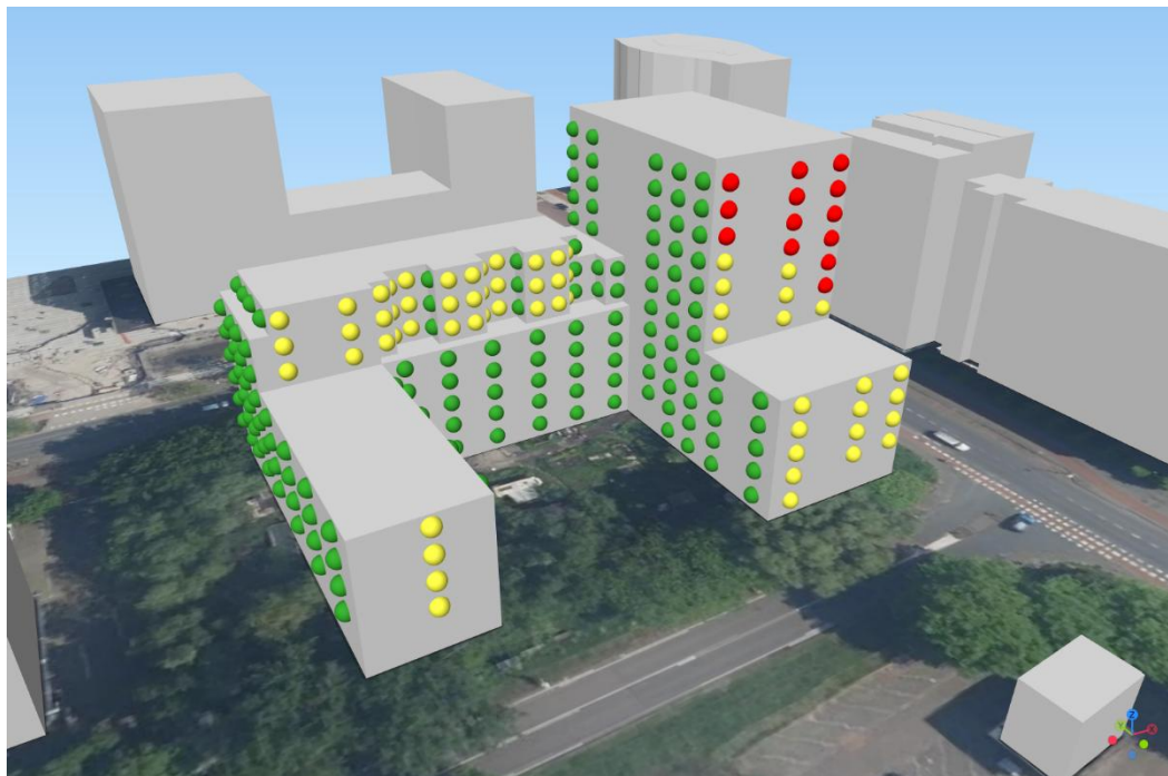
f 4.5 Geluid van rijkswegen
