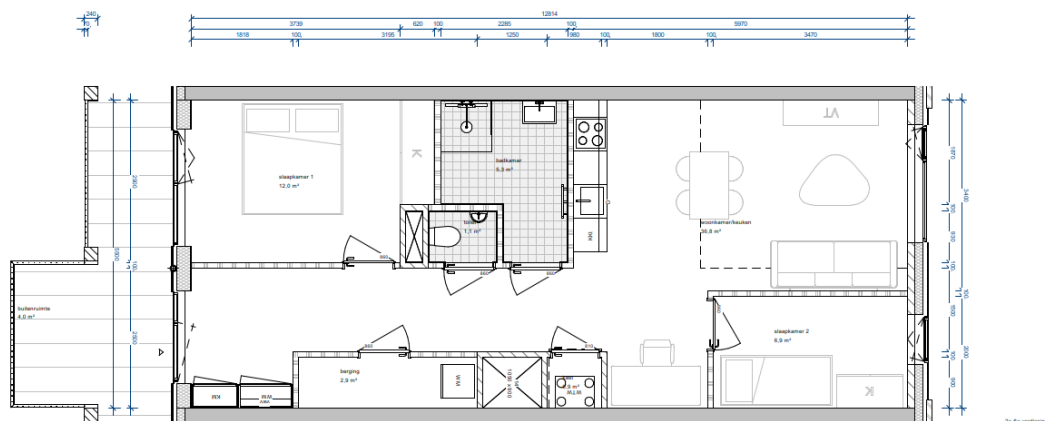
f 5.9 Woningtype B6 (plattegrond geroteerd)
