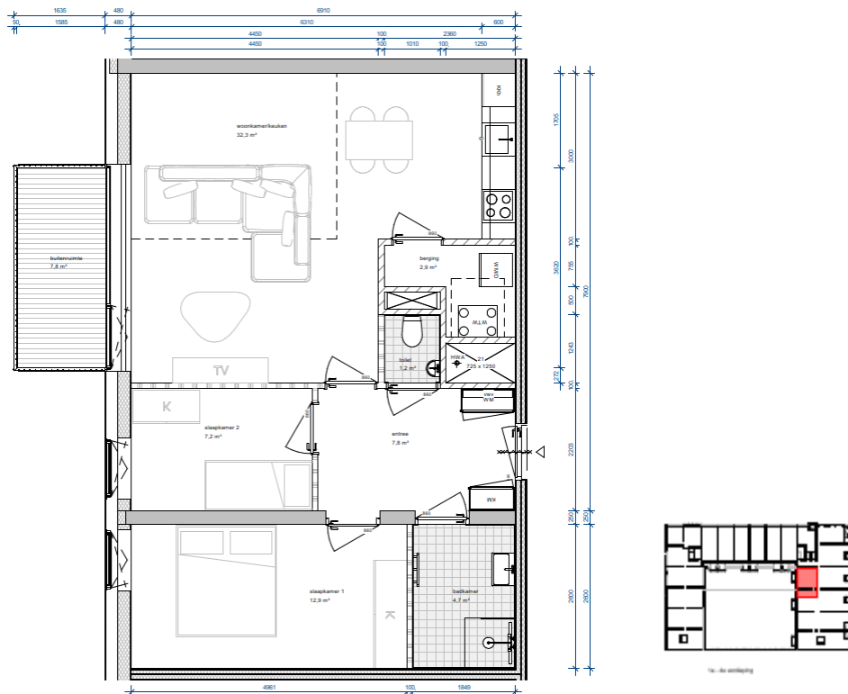
f 5.21 Woningtype C4
