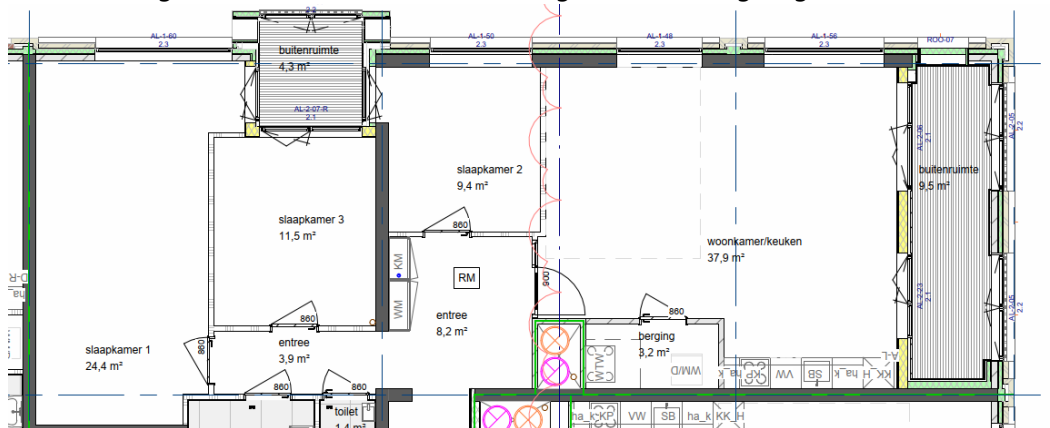
f 5.18 Woningtype C2
