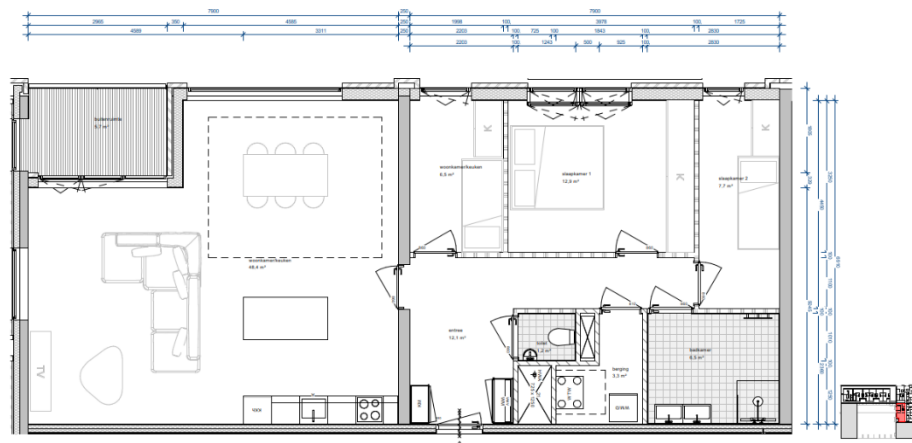
f 5.24 Woningtype C7 (plattegrond geroteerd)
