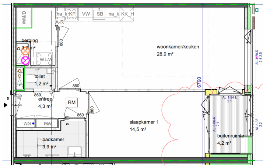
f 5.31 Woningtype D4
