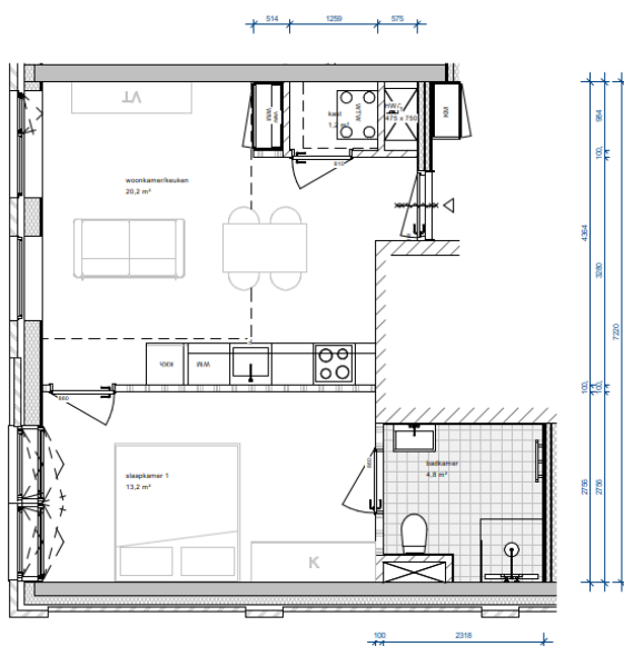
f 5.3 Woningtype A2
