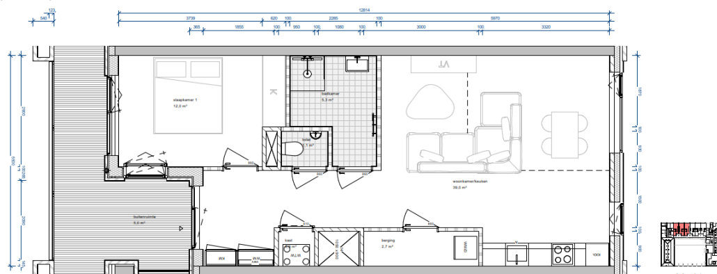
f 5.11 Woningtype B7 (plattegrond geroteerd)
