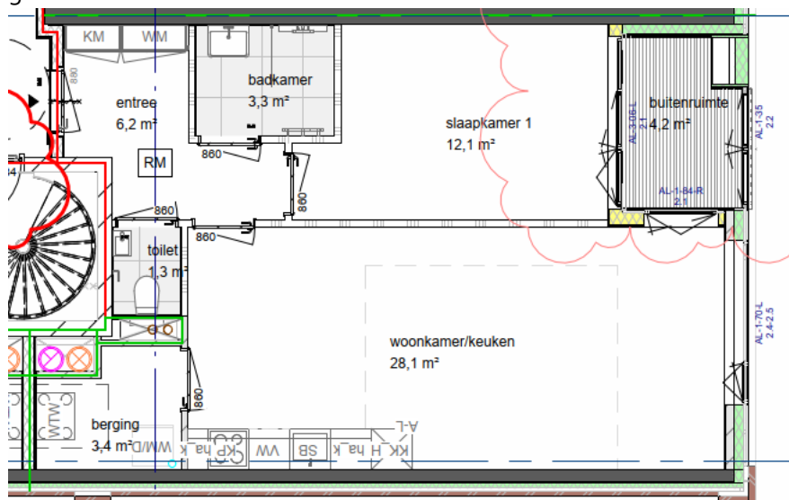
f 5.32 Woningtype D5
