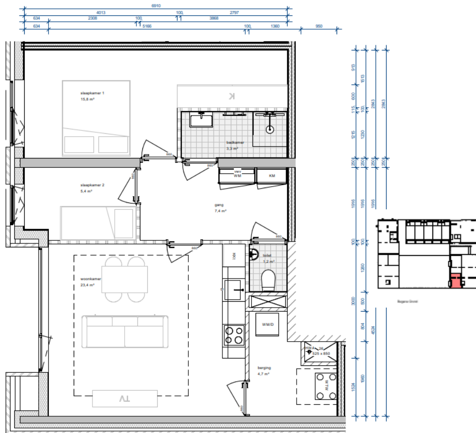
f 5.27 Woningtype D1
