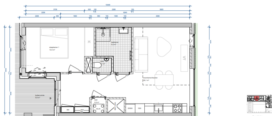
f 5.13 Woningtype B8 (plattegrond geroteerd)
