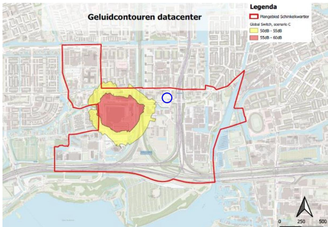
f 2.9 Geluidcontouren Global Switch (op 30 meter hoogte), zoals gepresenteerd in het Omgevingseffectrapport Schinkelkwartier.
