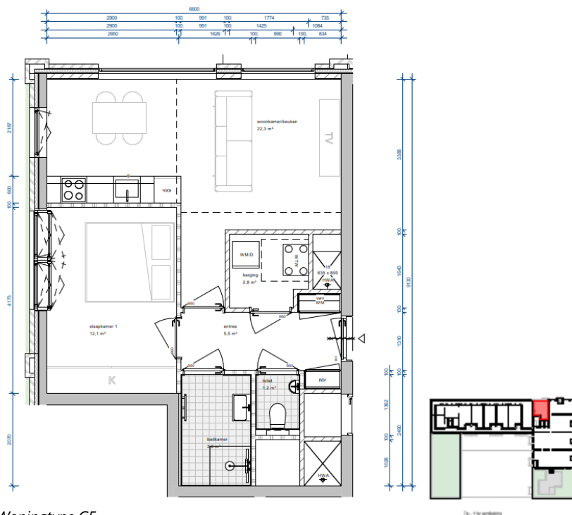
f 5.22 Woningtype C5
