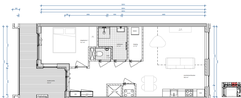
f 5.12 Woningtype B7* met niet-geluidgevoelige noordgevel (plattegrond geroteerd)
