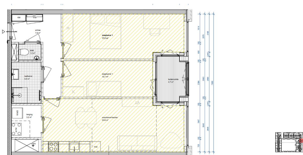
f 5.20 Woningtype C3**
