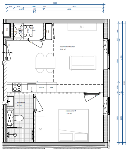
f 5.2 Woningtype A1
