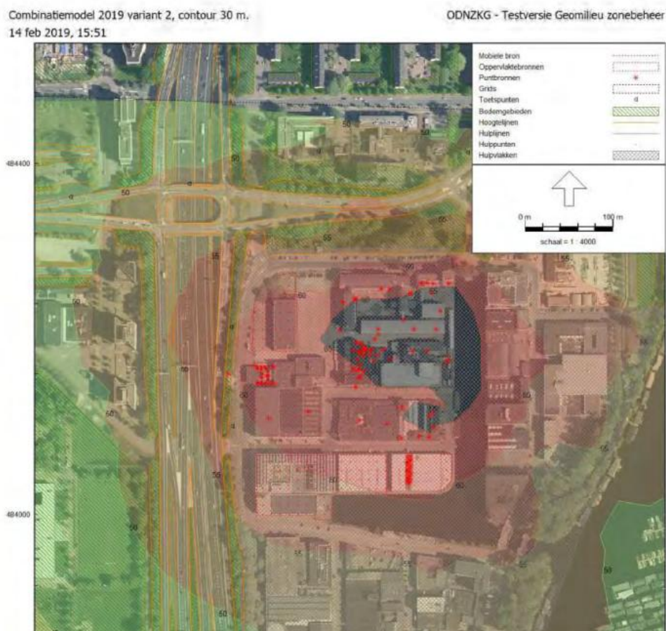
f 2.7 Geluidcontouren industrieterrein Schinkel op 30 meter hoogte, variant 2.
