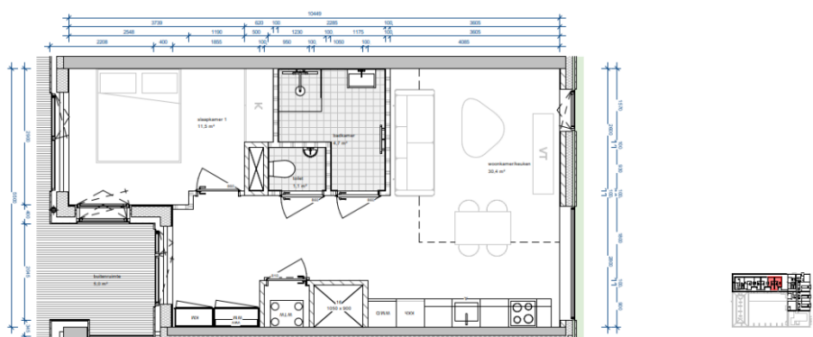
f 5.14 Woningtype B8* (plattegrond geroteerd)
