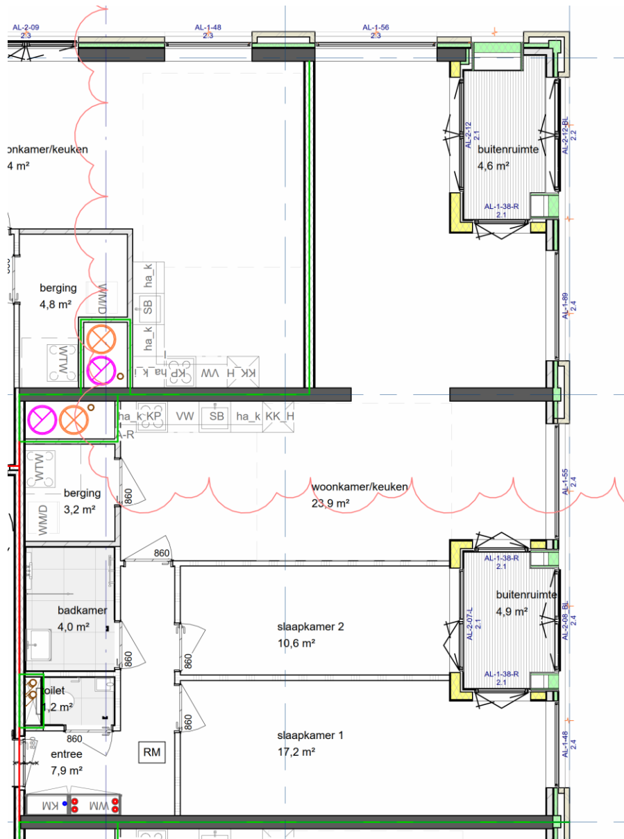
f 5.26 Woningtype C9
