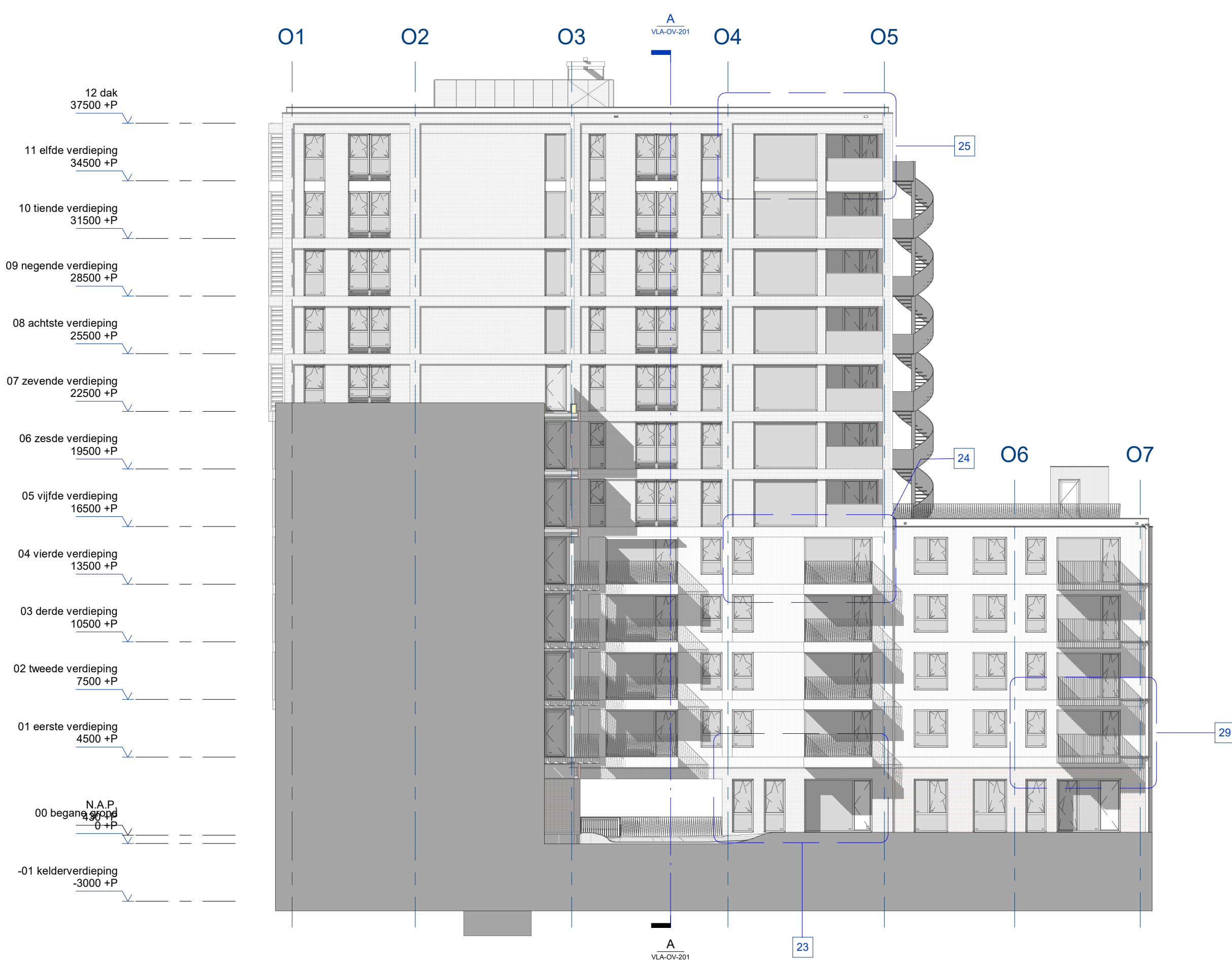
binnengevel west_Fragmenten schaal 1 : 200
