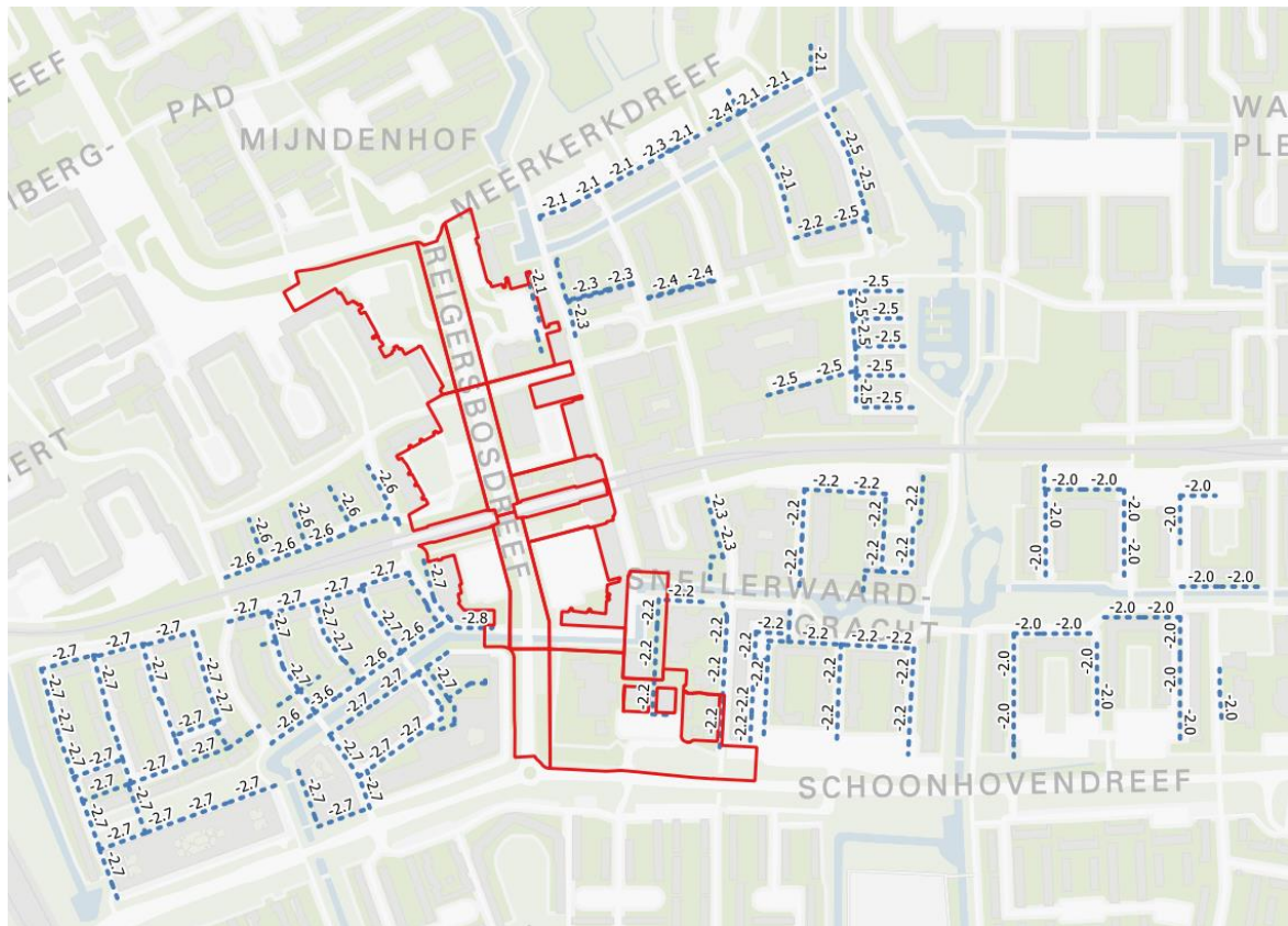
Figuur 2-8 Aanwezige drainage met buishoogte (B.O.B.) [m +NAP] (Riolering Waternet)
