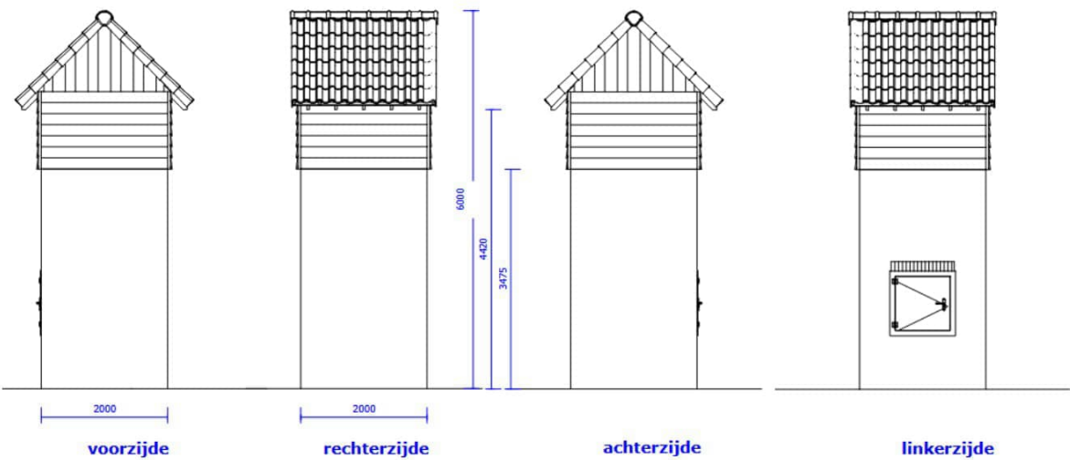
aanzichten 1:50
