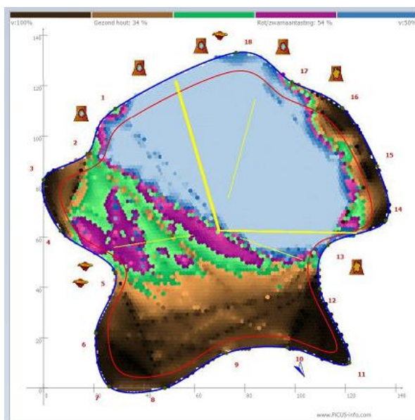
Het tomogram laat een zeer omvangrijke rotting zien. Deze komt overeen met de prikstok controle. Het blauwe deel is zeer zwaar aangetast hout. Over meer dan 60% van de omtrek is er onvoldoende restwand. Gezien de hoogte van de boom is er een zeer hoog risico op stambreuk. De boom kan niet gehandhaafd worden.
