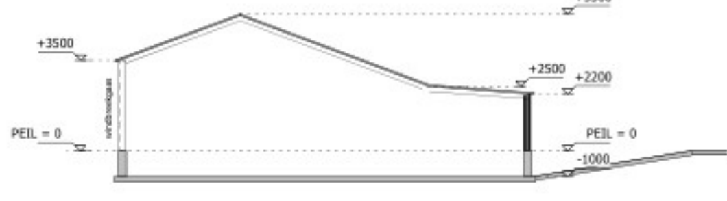
DOORSNEDE GEBOUW 3B
