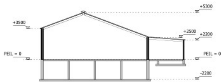
DOORSNEDE GEBOUW 3A
