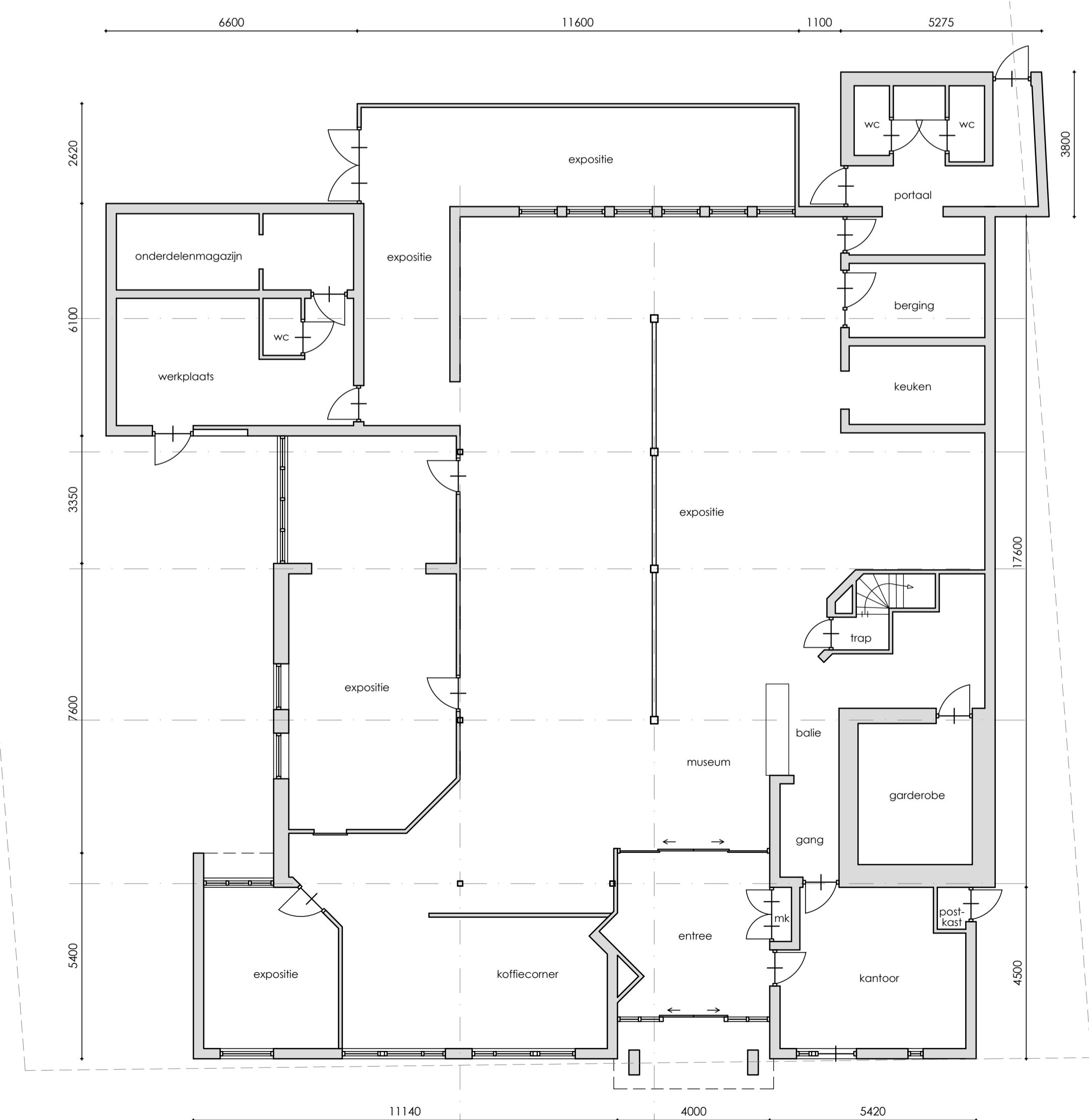
BEGANE GROND BESTAAND
