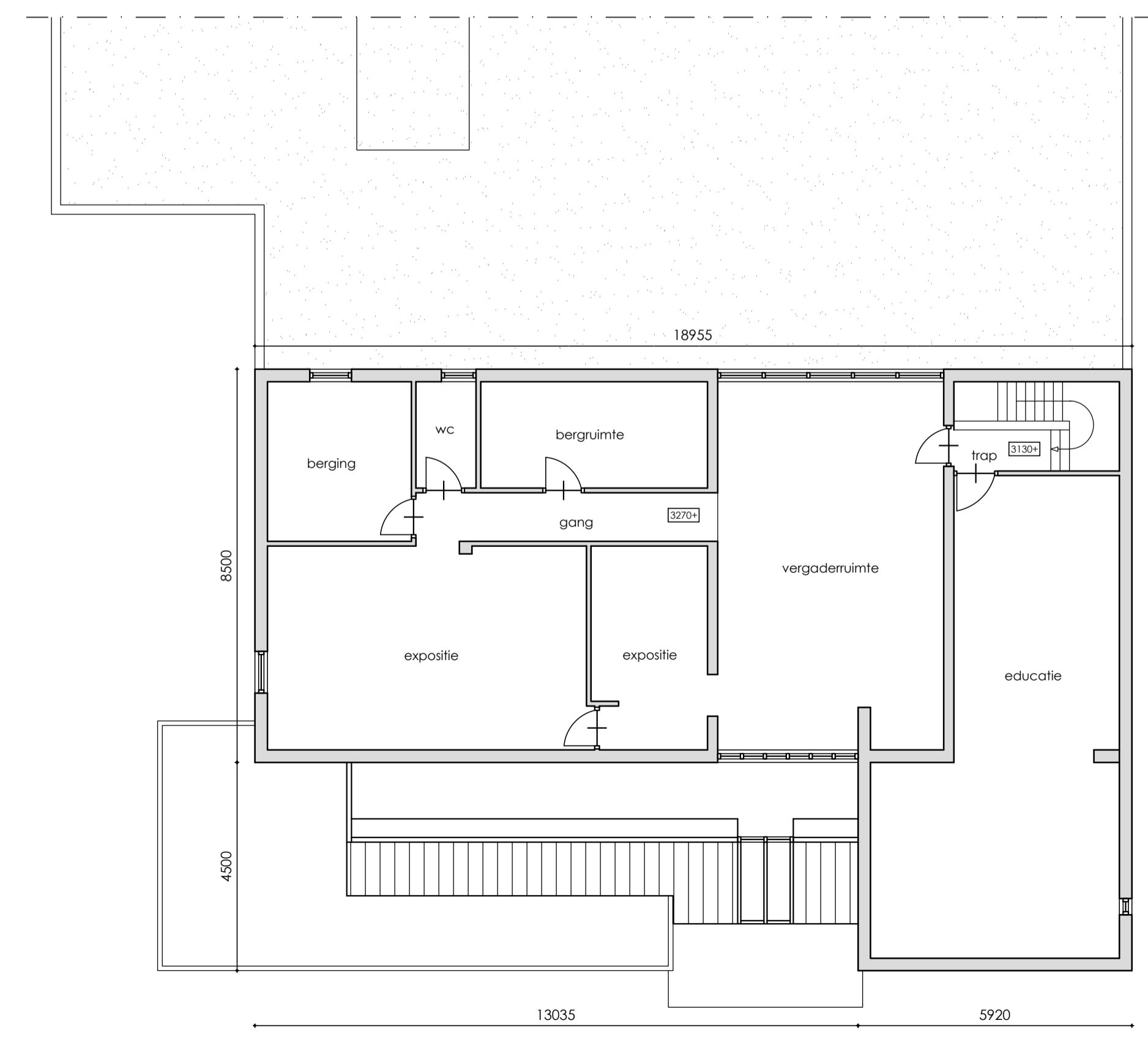
VERDIEPING BESTAAND
