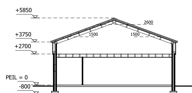
DOORSNEDE GEBOUW 1
