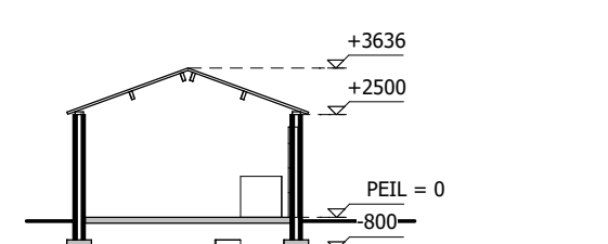
DOORSNEDE GEBOUW 4
