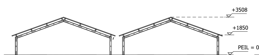
DOORSNEDE GEBOUW 6
