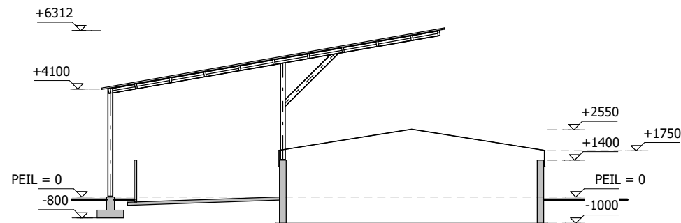
DOORSNEDE GEBOUW 3
