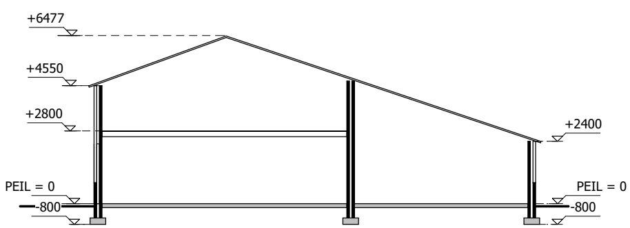
DOORSNEDE GEBOUW 2
