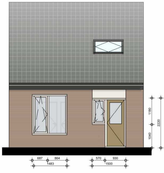
Achtergevel
