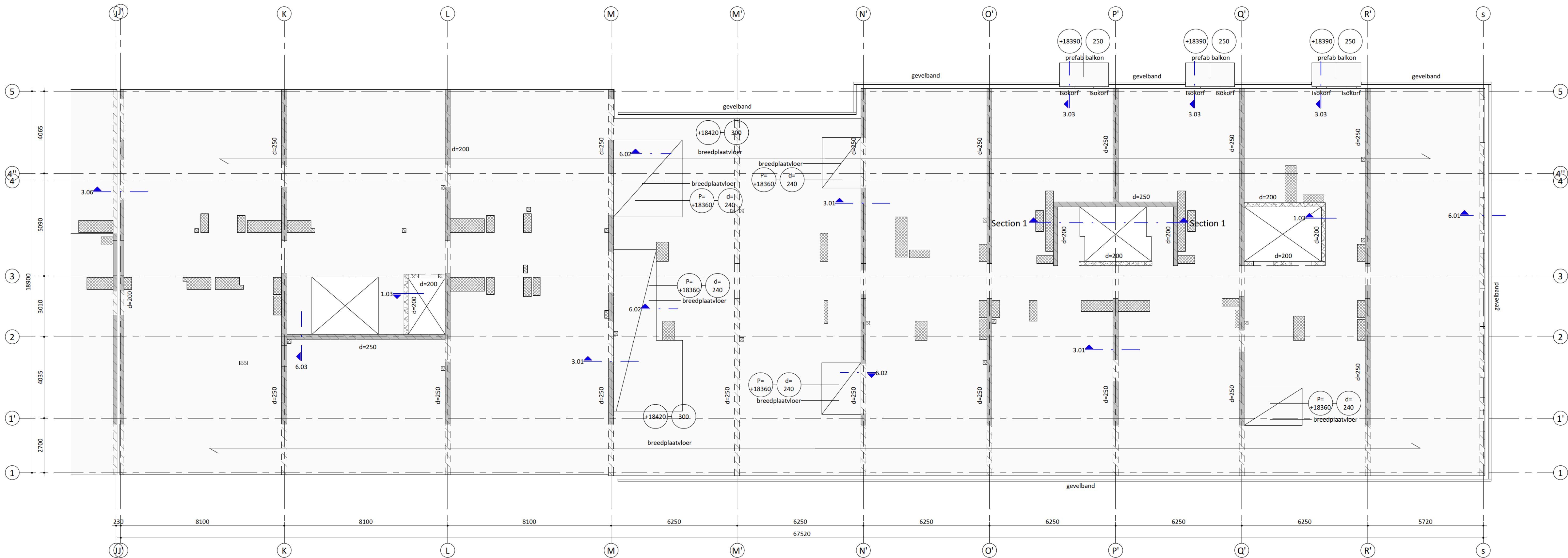
zesde verdieping 1 : 100
