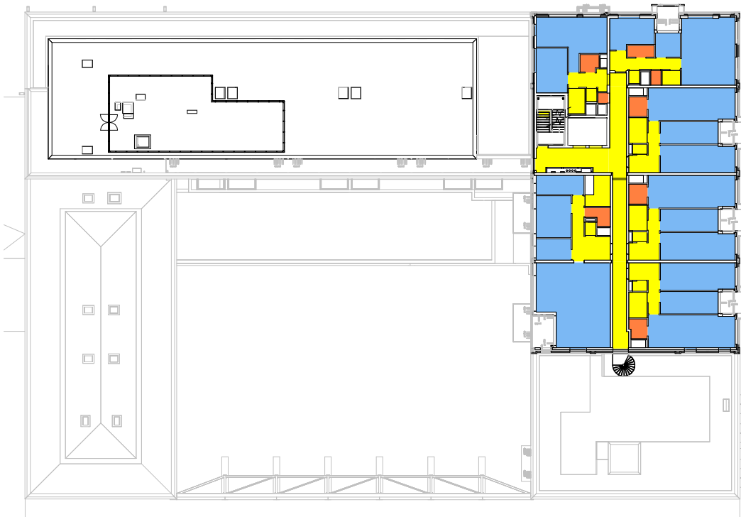
08 achte verdieping schaal 1 : 500
