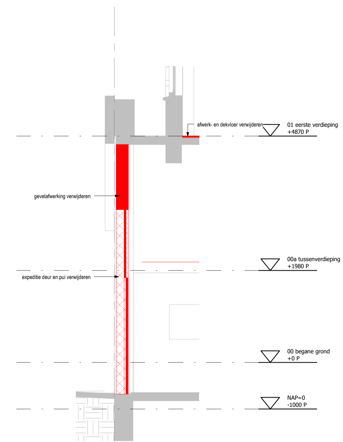
03_doorsneden_fragment 1_2_A1_05_A
