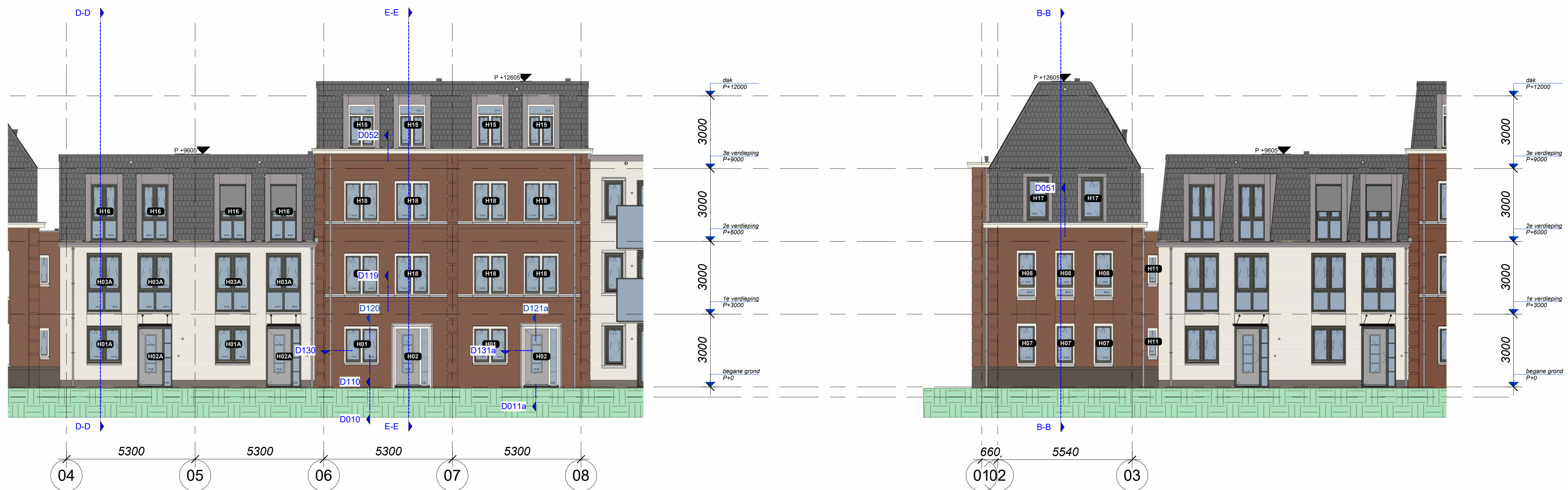
voorgevel BNR 2-3-4-5 (Westgevel) 1 : 100
