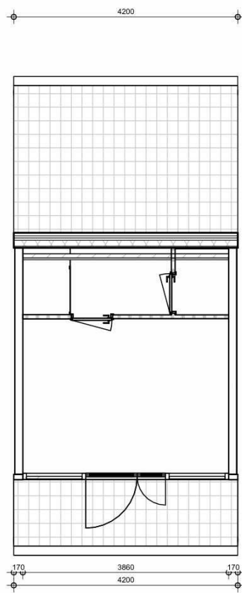
eerste verdieping
