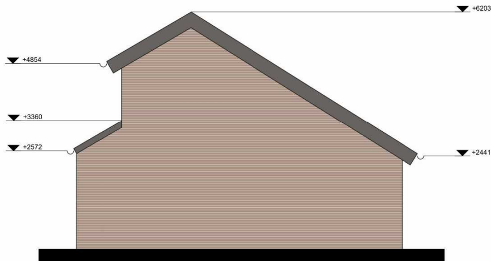
Zijgevel
