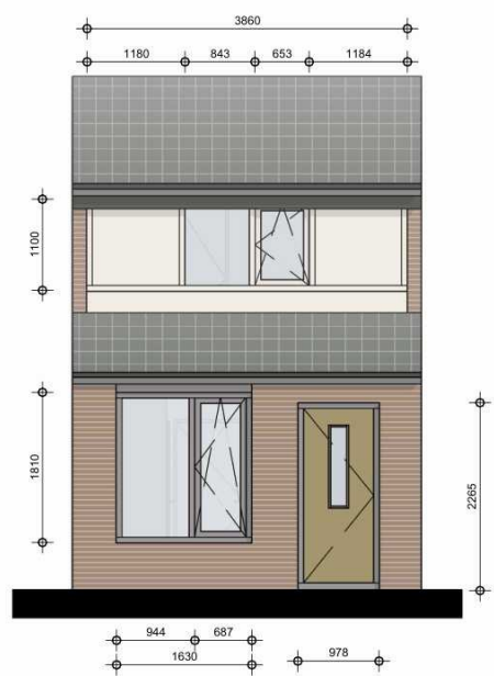
Voorgevel
