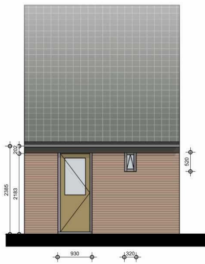
Achtergevel
