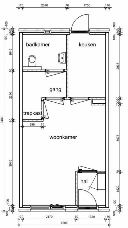
begane grond
