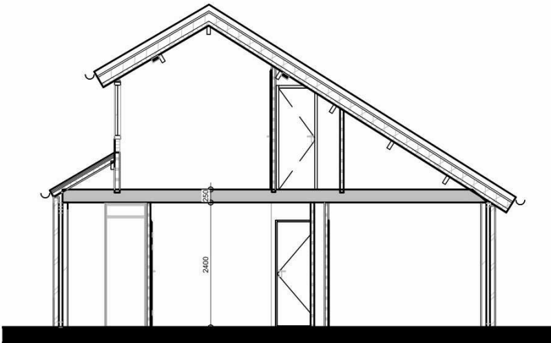
B-B
