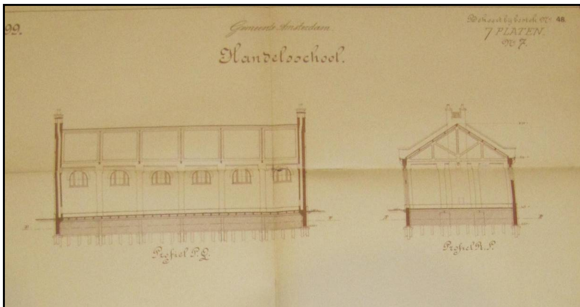
Afb. 28. Deel van een ontwerptekening uit 1899, met daarop de kapconstructie van het gymnastiekgebouw.
