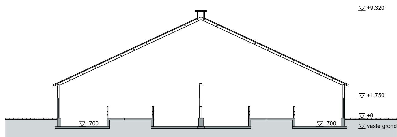
Doorsnede B-B
