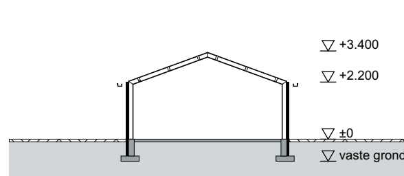
Doorsnede G-G
