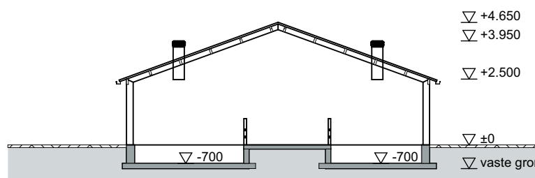
Doorsnede D-D
