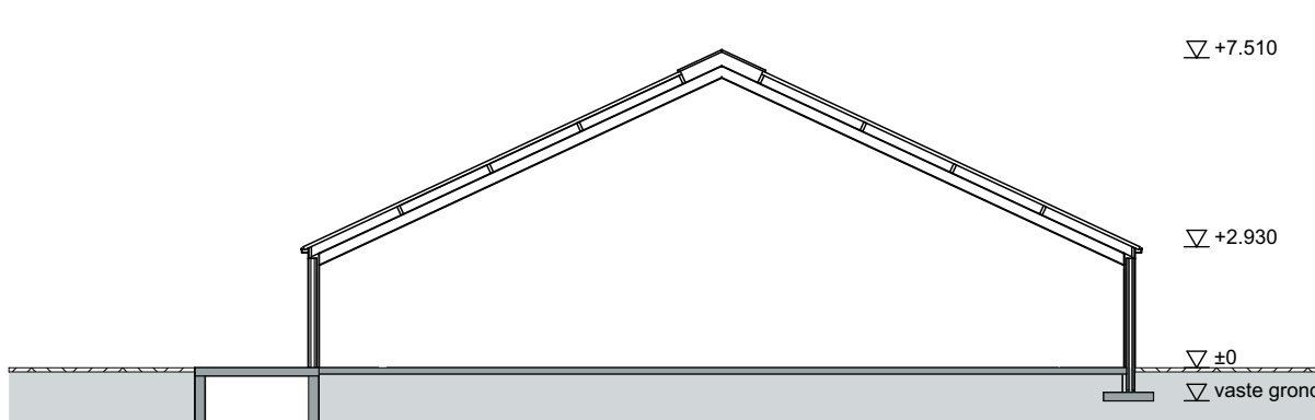
Doorsnede H-H
