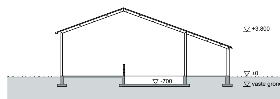
Doorsnede C-C
