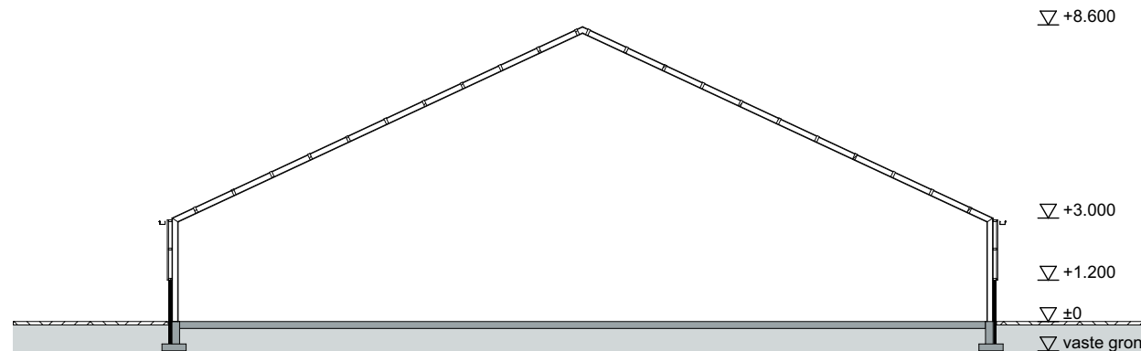
Doorsnede F-F
