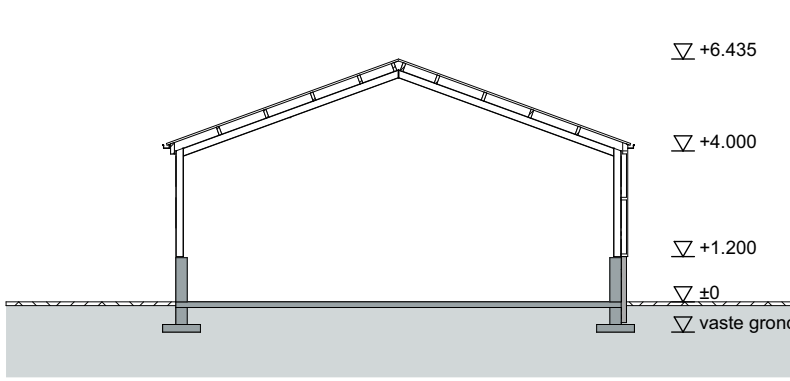
Doorsnede E-E
