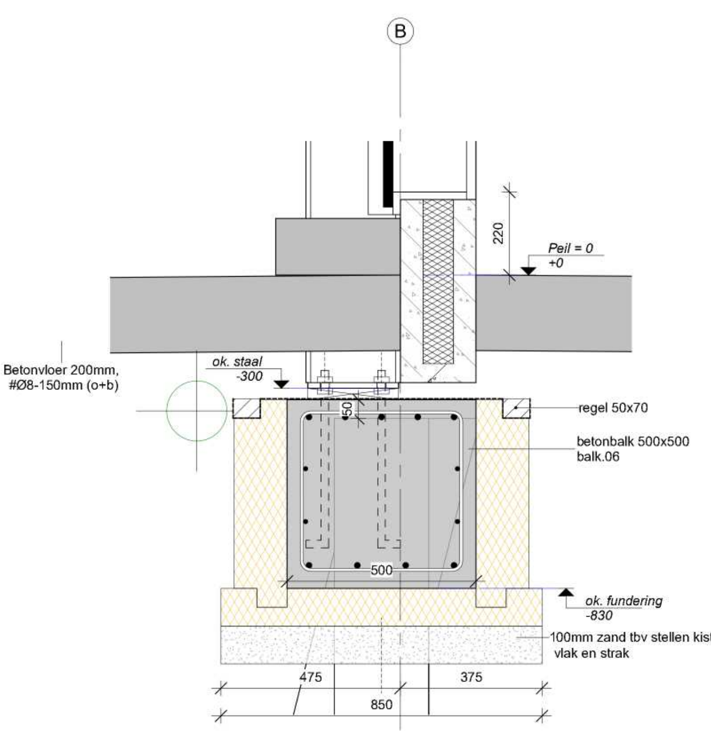
Detail 1.2 linker zijgevel - Fund 1 : 10
