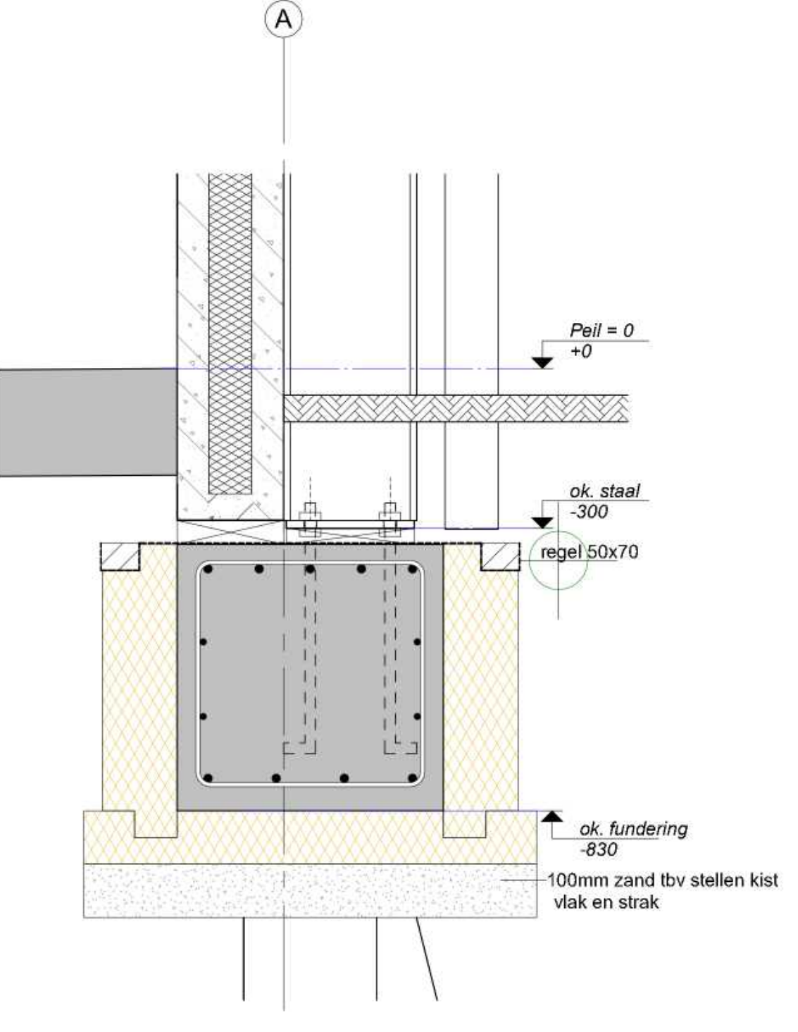
Detail 1.1 rechter zijgevel - Fund 1 : 10
