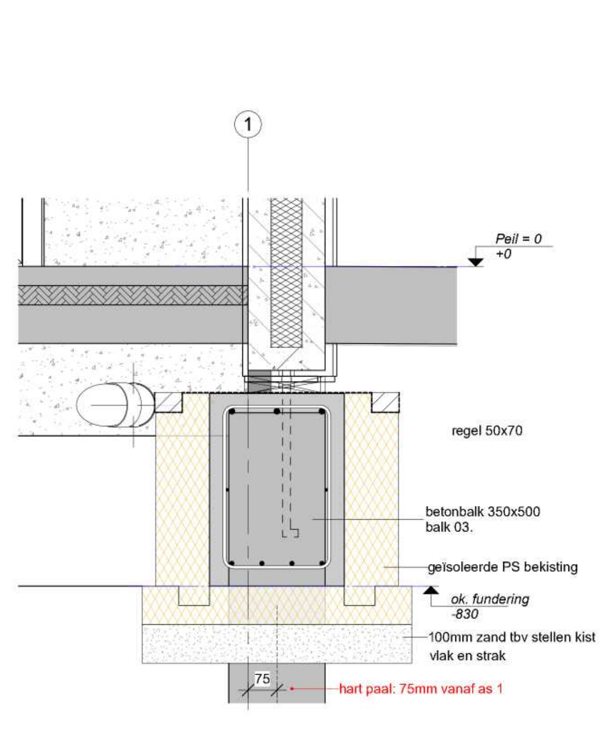
Detail 2.1 kopgevel - Fund 1 : 10
