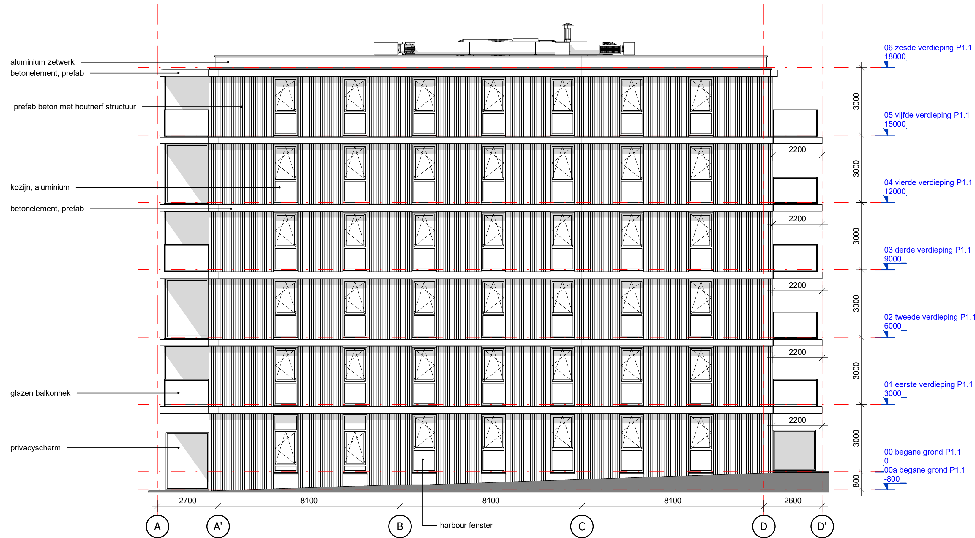
Zuidgevel
