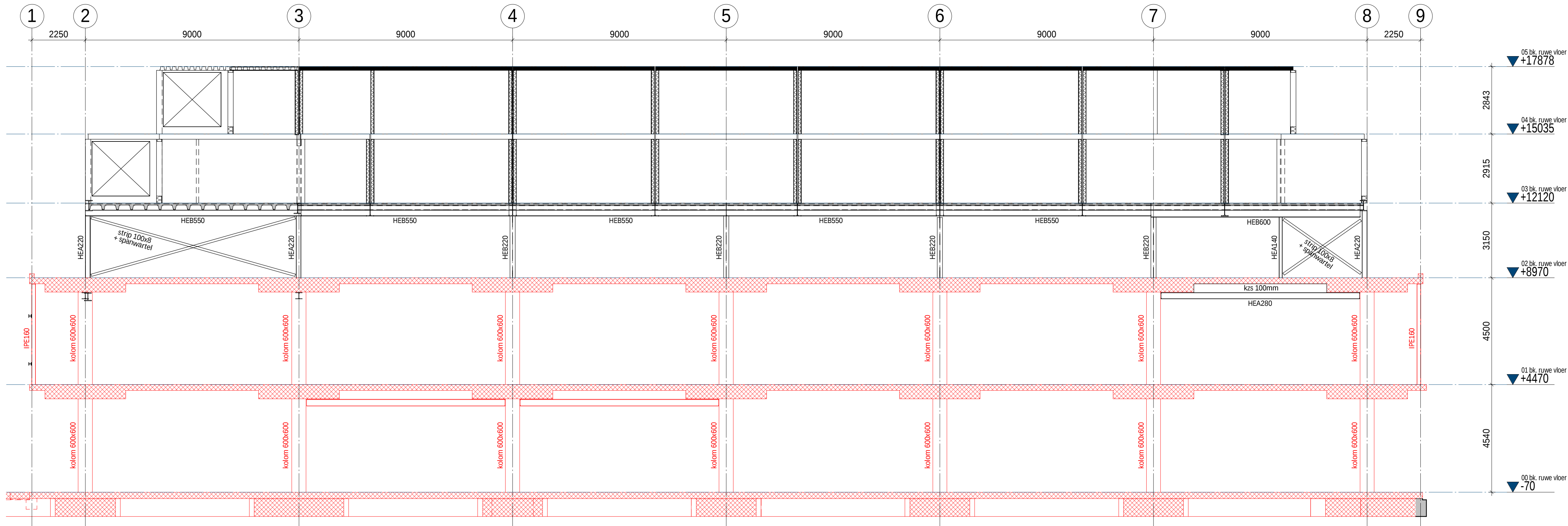
Aanzicht as C 1 : 100
