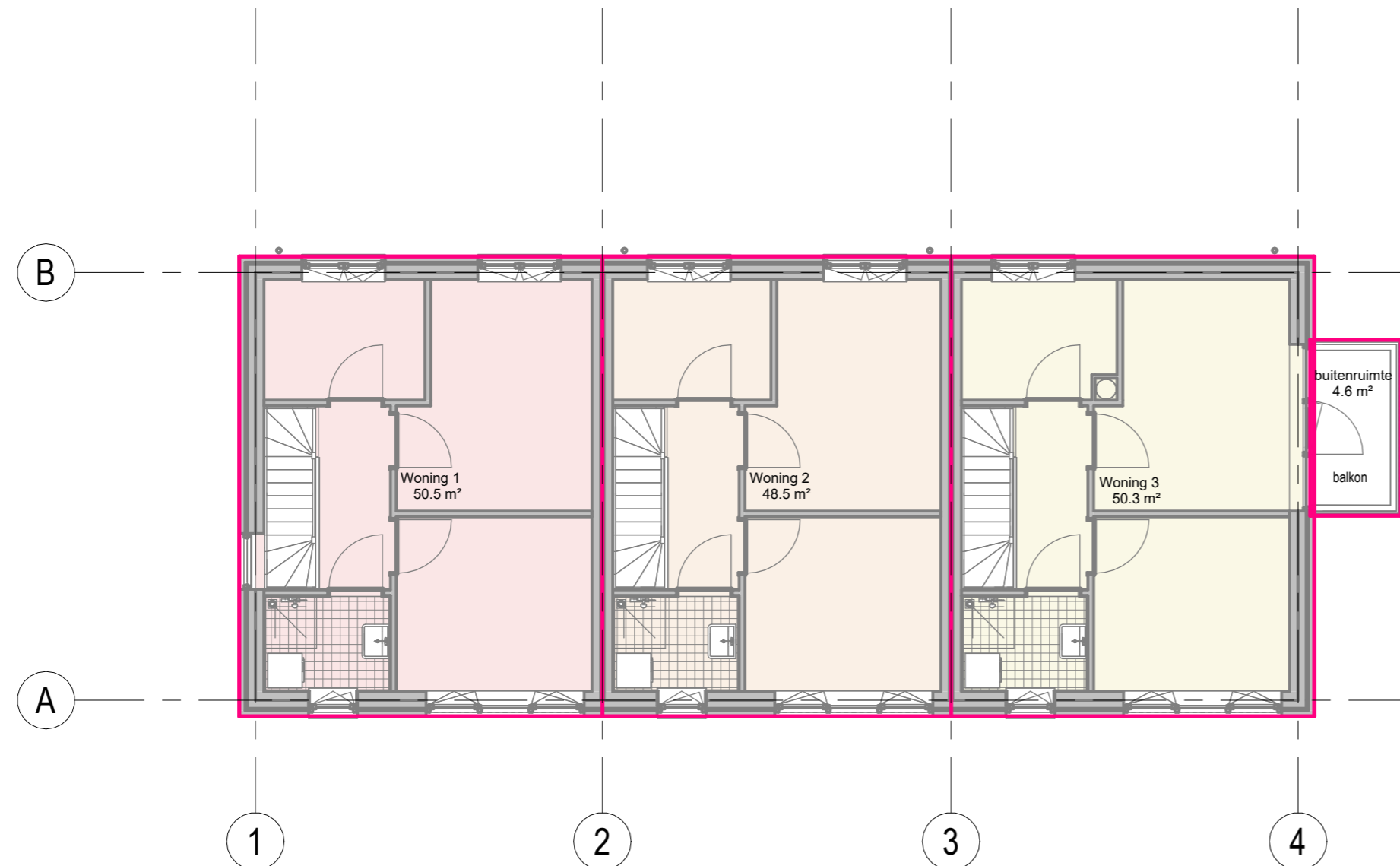
Eerste verdieping 1 : 100
