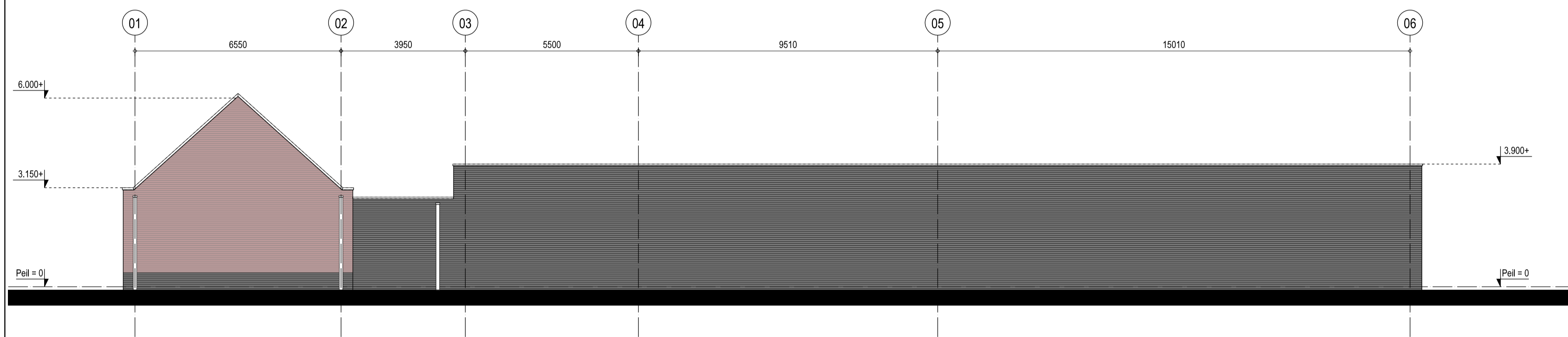
Rchtergevel
