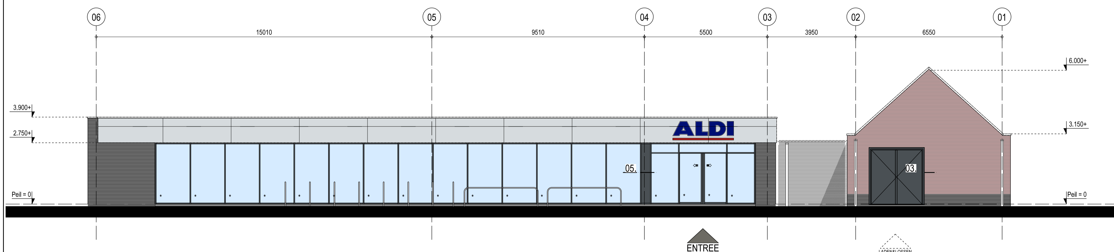
Linker zijgevel
